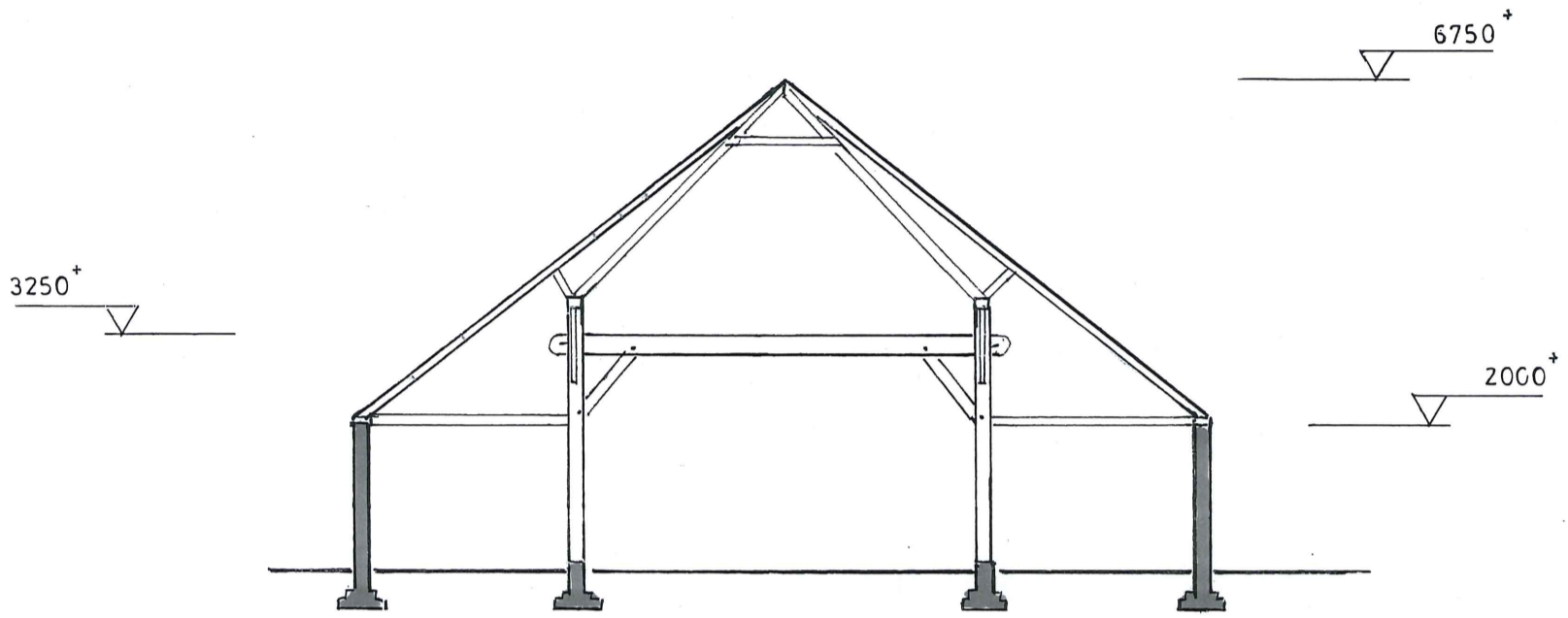
Doorsnede A-A
