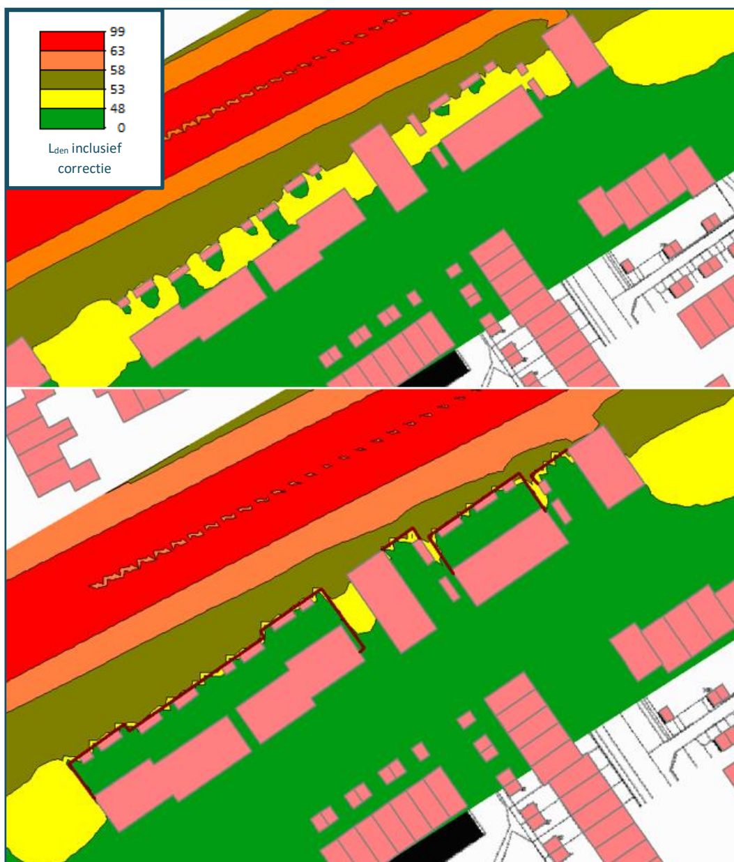
Figuur 11 Weergave van de geluidsbelasting 1,5 meter hoogte in de tuinen op het westelijke blok vanwege de Broekheurnering voor het plaatsen van een tuinschermen (boven) en na het plaatsen van tuinschermen (onder)
