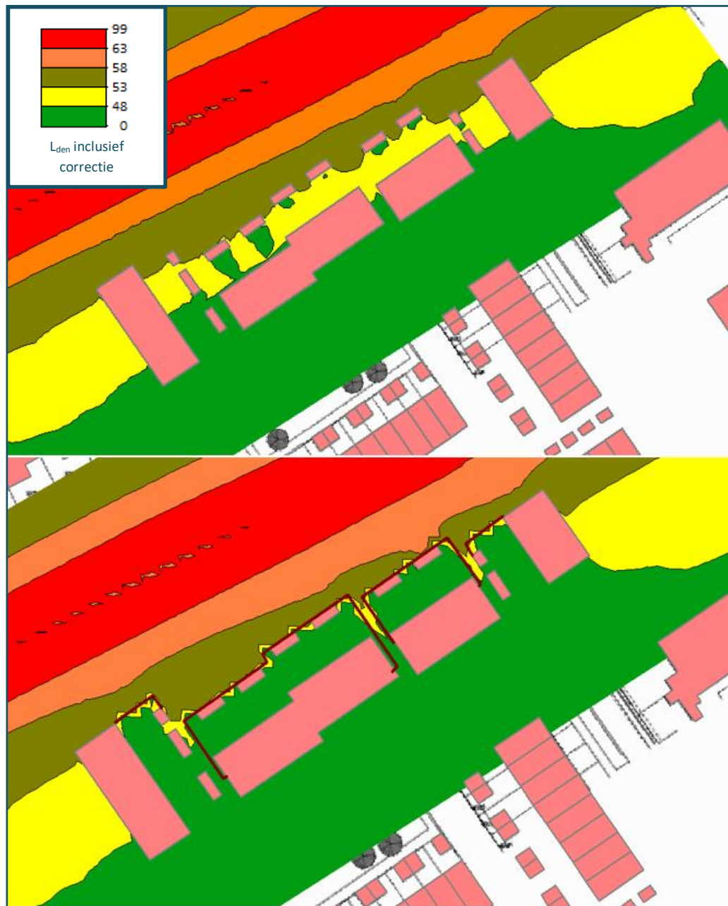
Figuur 10 Weergave van de geluidsbelasting op 1,5 meter hoogte in de tuinen op het oostelijke blok vanwege de Broekheurnering voor het plaatsen van tuinschermen (boven) en na het plaatsen van tuinschermen (onder)
