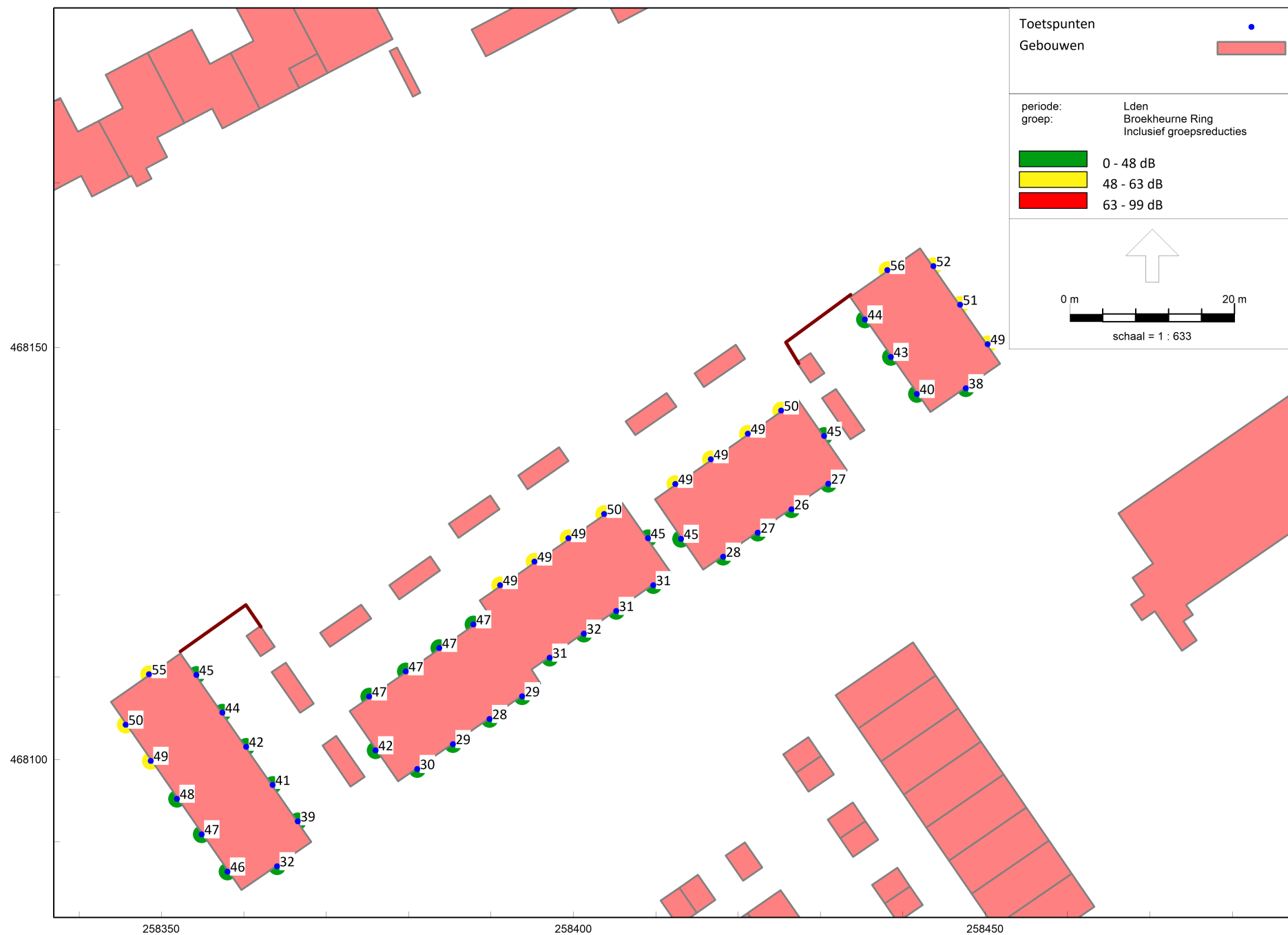
Figuur 7 Geluidsbelasting vanwege wegverkeer op de Broekheurnering inclusief 5 dB correctie t.b.v geluidluw geveldeel
