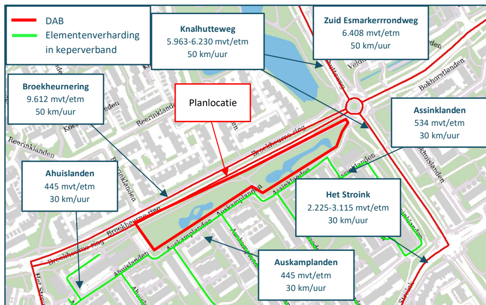
Figuur 2 Verkeers- en verhardingsgegevens lokale wegen 2032
