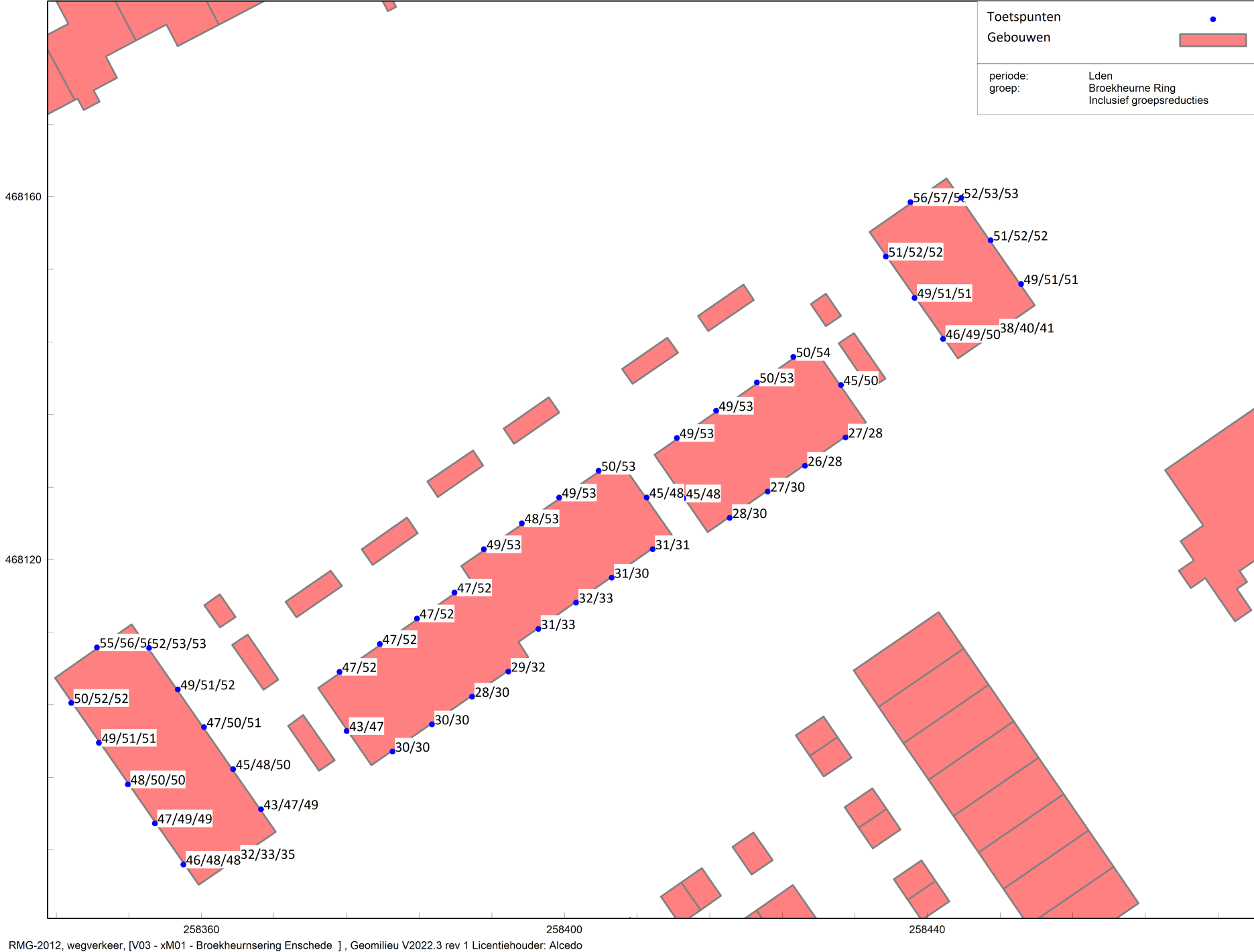
Figuur 5 Geluidsbelastingen vanwege wegverkeer op de Broekheurnering inclusief 5 dB correctie conform artikel 110g Wgh (oostelijk blok)
