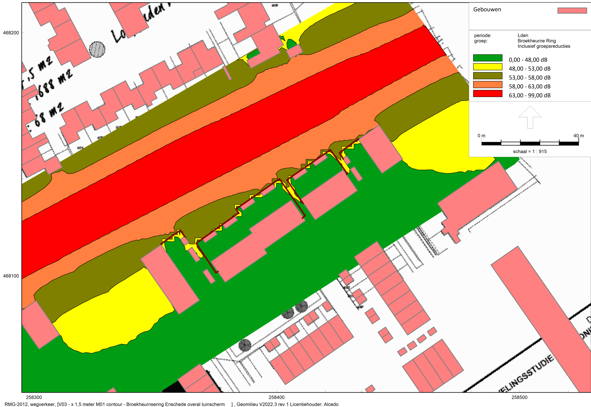
Figuur 11 Contourberekening (1,5 meter beoordelingshoogte) oostelijk blok
