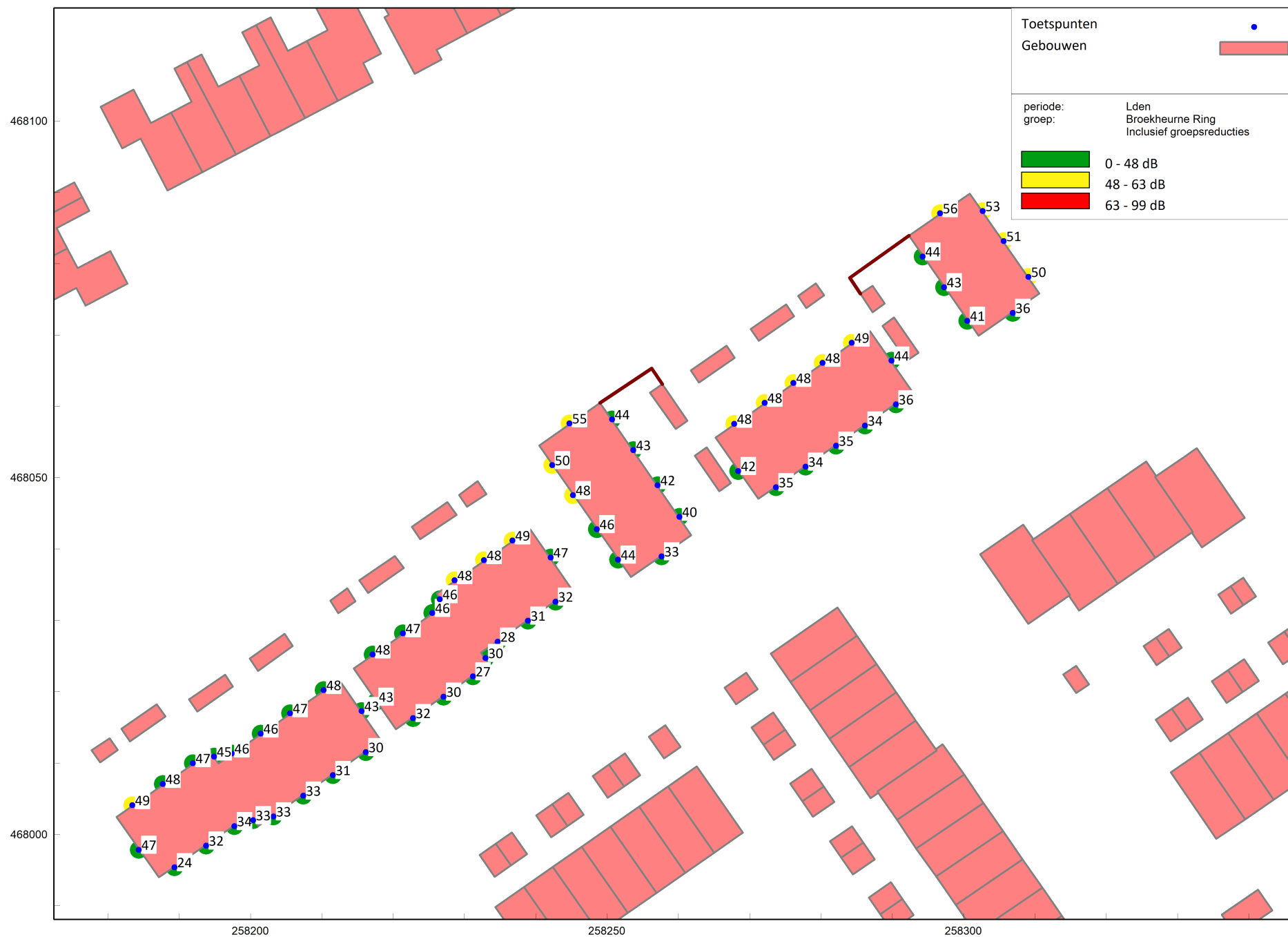
Figuur 8 Geluidsbelasting vanwege wegverkeer op de Broekheurnering inclusief 5 dB correctie t.b.v geluidluw geveldeel
