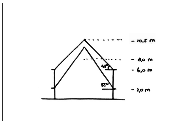
Figuur 32 Dakhelling boerderijwoning ligt tussen de 45 graden en 55 graden. Bouwhoogte boerderijwoning ligt tussen 8,0 en 10,5 meter. Goothoogte boerderijwoning ligt tussen de 2,0 en 6,0 meter.
