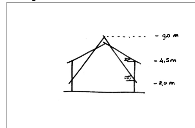
Figuur 40 Dakhelling beheergebouw ligt tussen 30 en 55 graden. Bouwhoogte beheergebouw is maximaal 9,0 meter. Goothoogte beheergebouw ligt tussen 2,0 en 4,5 meter.
