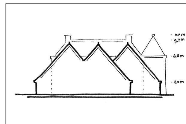
Figuur 23 Globale afmetingen profiel huidige ontwerp boerderij van allure.
