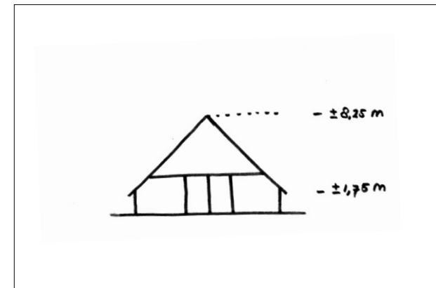
Figuur 24 Globale afmetingen profiel schuilkerk.
