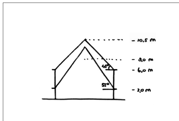
Figuur 25 Dakhelling schuurwoning ligt tussen de 45 graden en 55 graden. Bouwhoogte schuurwoning ligt tussen 8,0 en 10,5 meter. Goothoogte schuurwoning ligt tussen de 2,0 en 6,0 meter.
