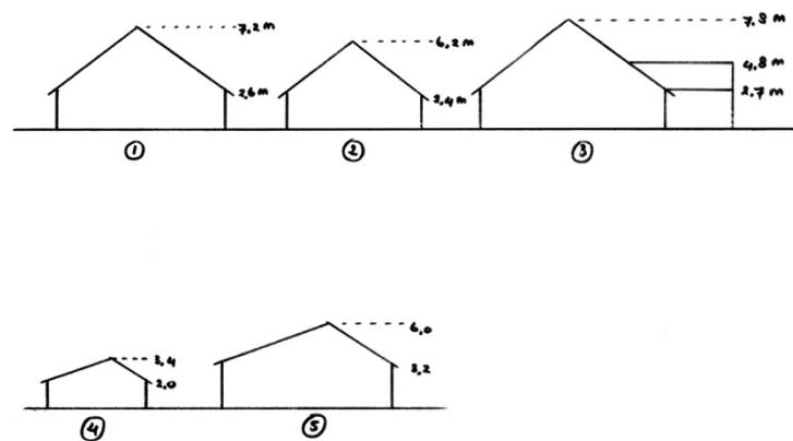
Figuur 38 Profielen van bestaande bebouwing Hokershoeve
