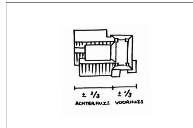
Figuur 21 Verhouding voor- en achterhuis boerderij van allure.
