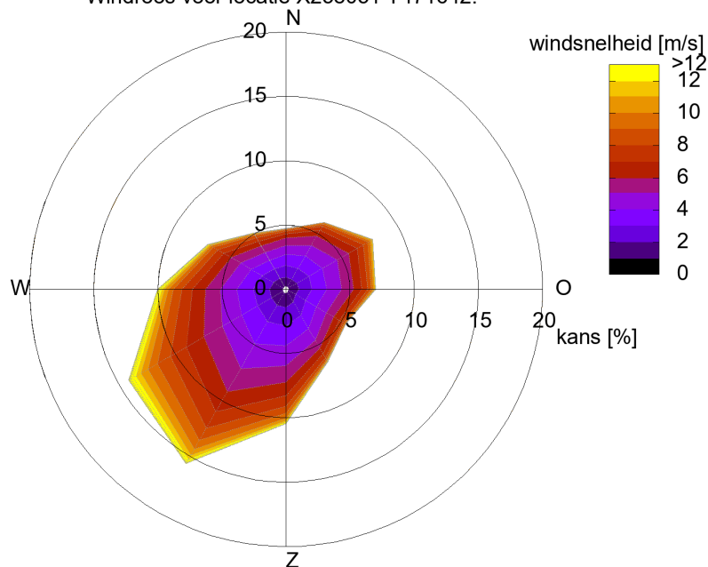
Windroos voor locatie X258051 Y471642.
