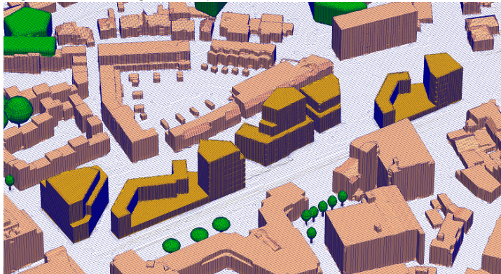
f3.2 Aanzicht oppervlakte grid rekenmodel, ingezoomd op het Pakhuis Kwartier
