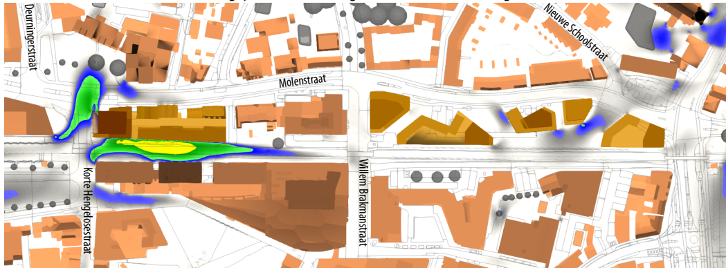
f3.3 Het te verwachten windklimaat in de geplande bebouwingssituatie, beoordeeld volgens de NEN 8100
