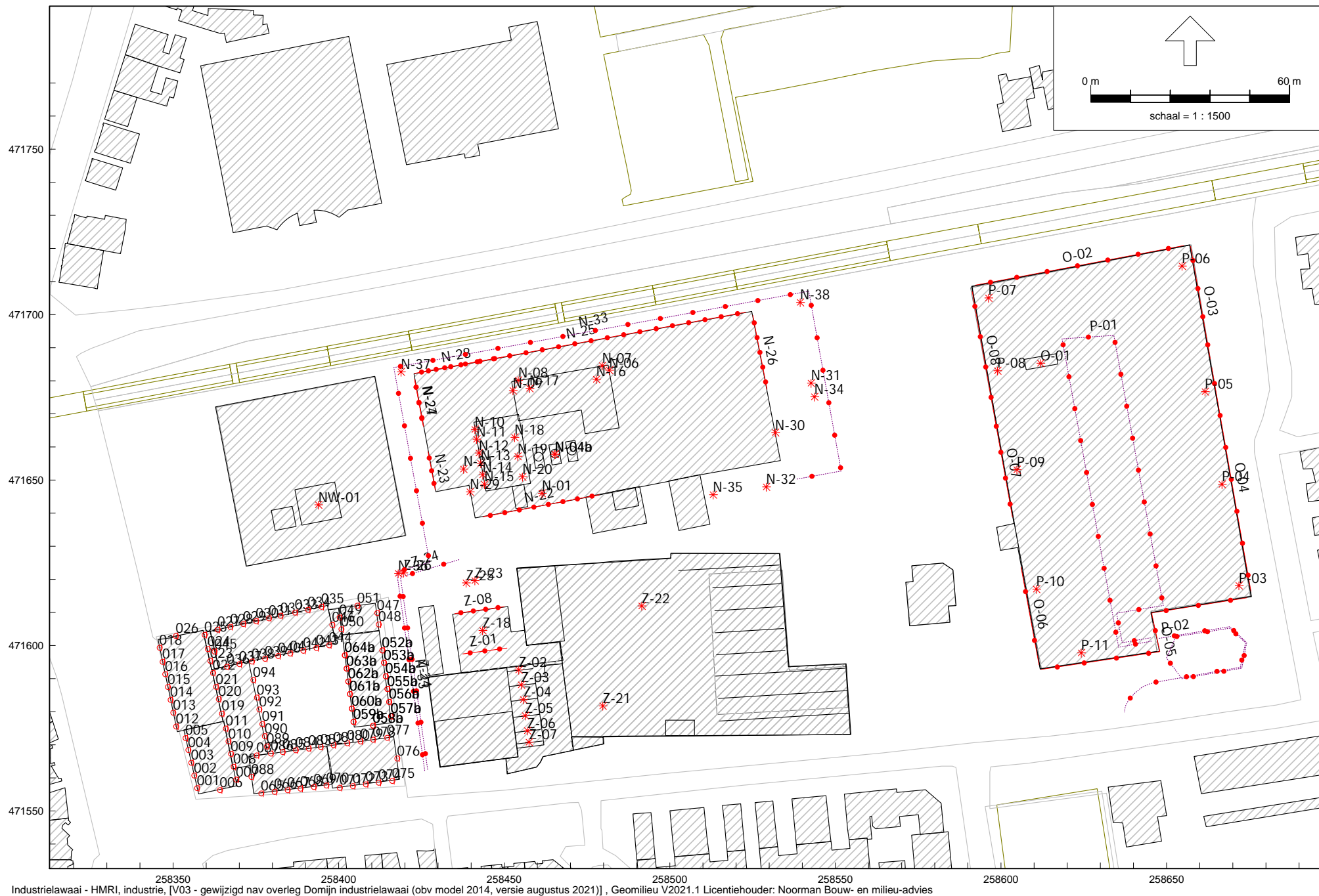
Overzicht geactualiseerd rekenmodel (industrielawaai)
