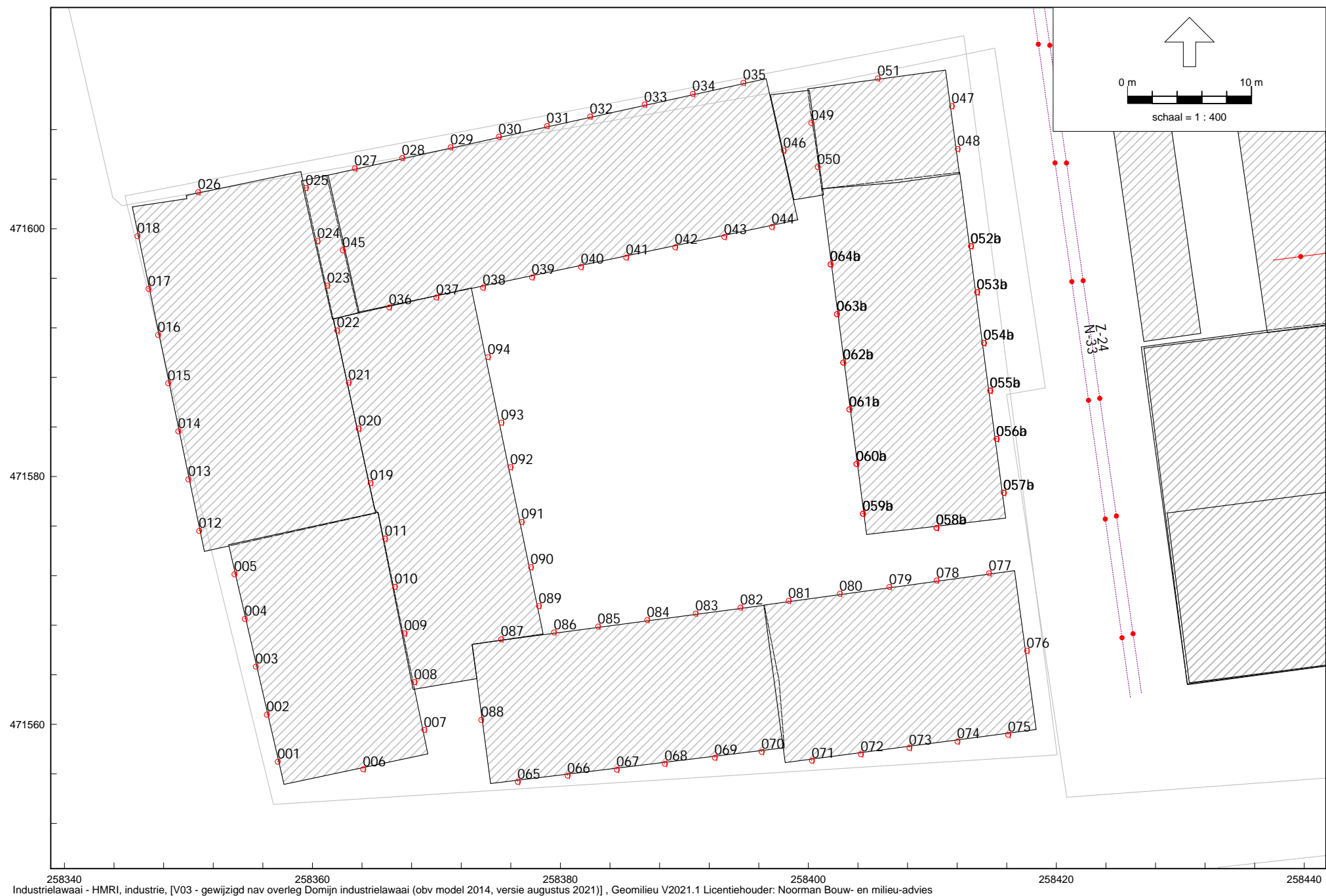
Overzicht geactualiseerd rekenmodel (industrielaawai) - detail rekenpunten
