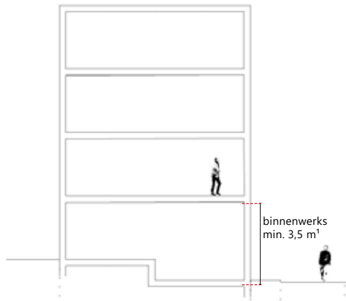
doorsnede Statenpanden langs de busbaan
