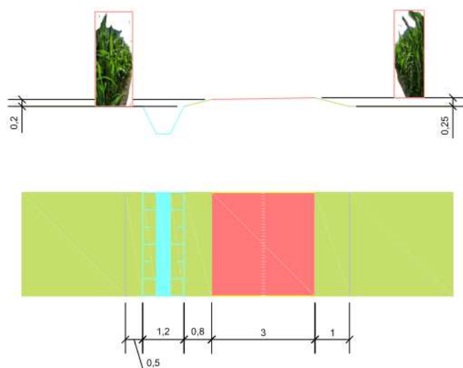
Doorsnede fietspad ter plaatse van doorsnijding agrarisch gebied
