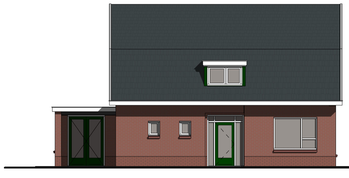
2 Linkergevel 1 : 100
