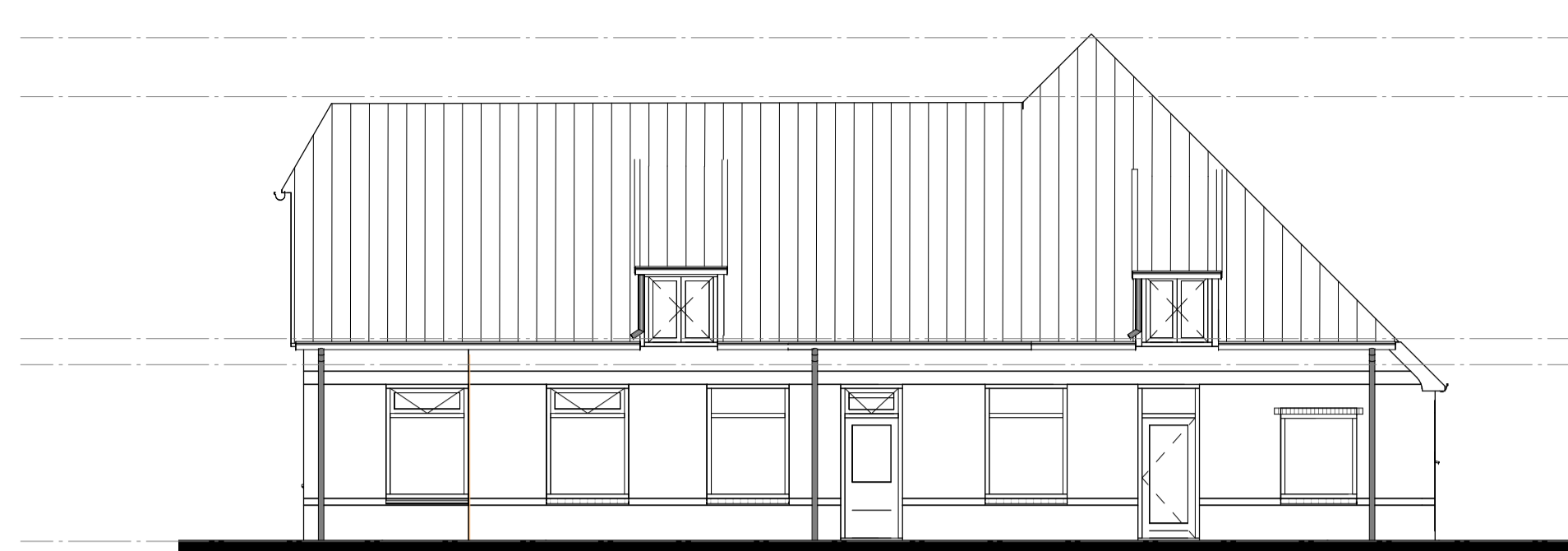
Voorgevel
