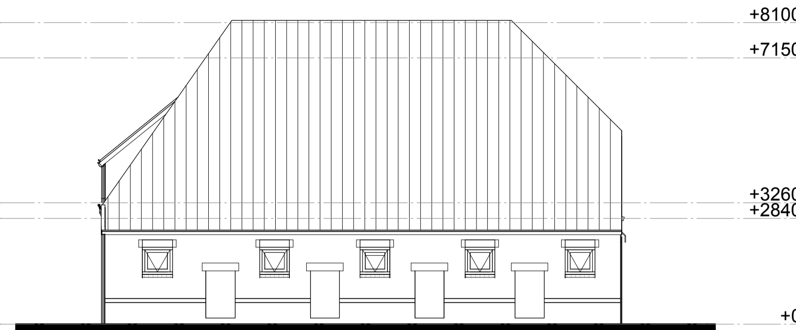
Rechtergevel
