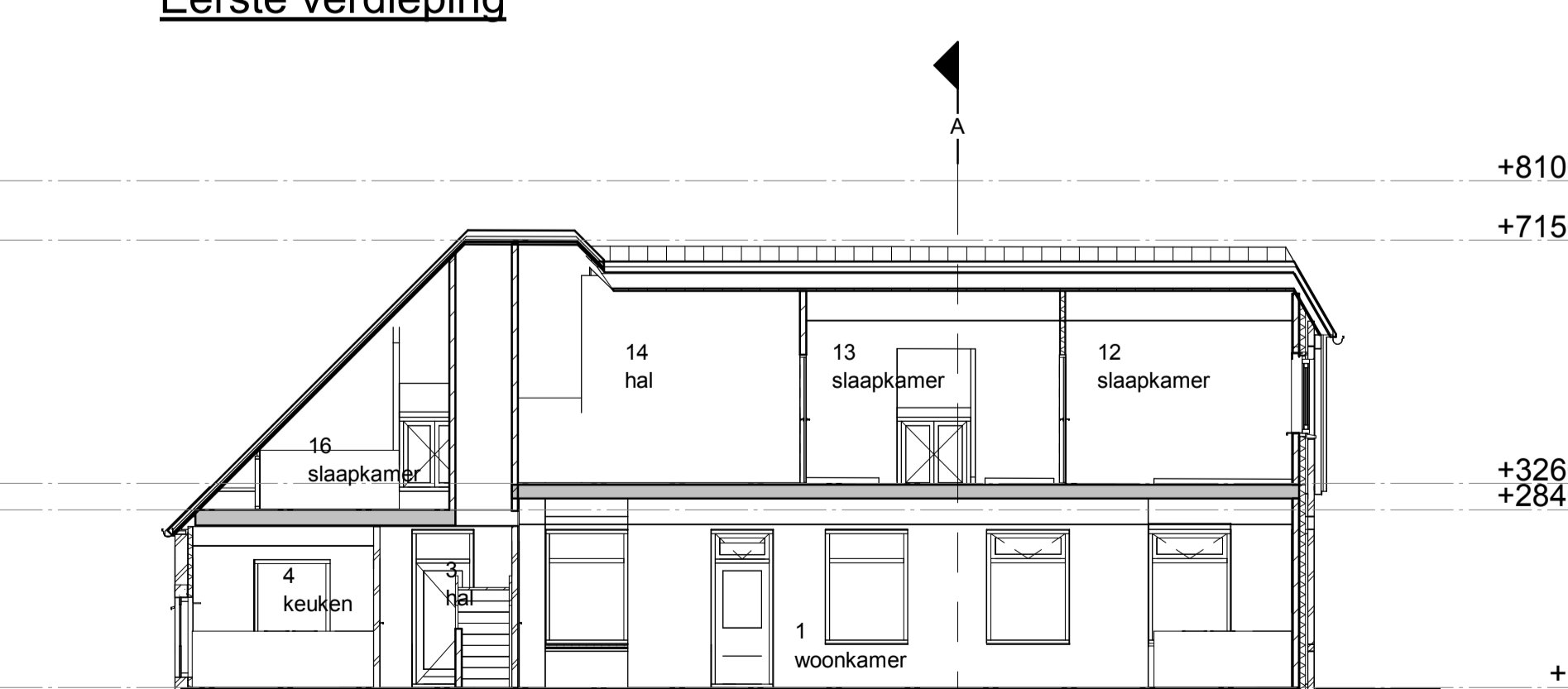
Doorsnede B
