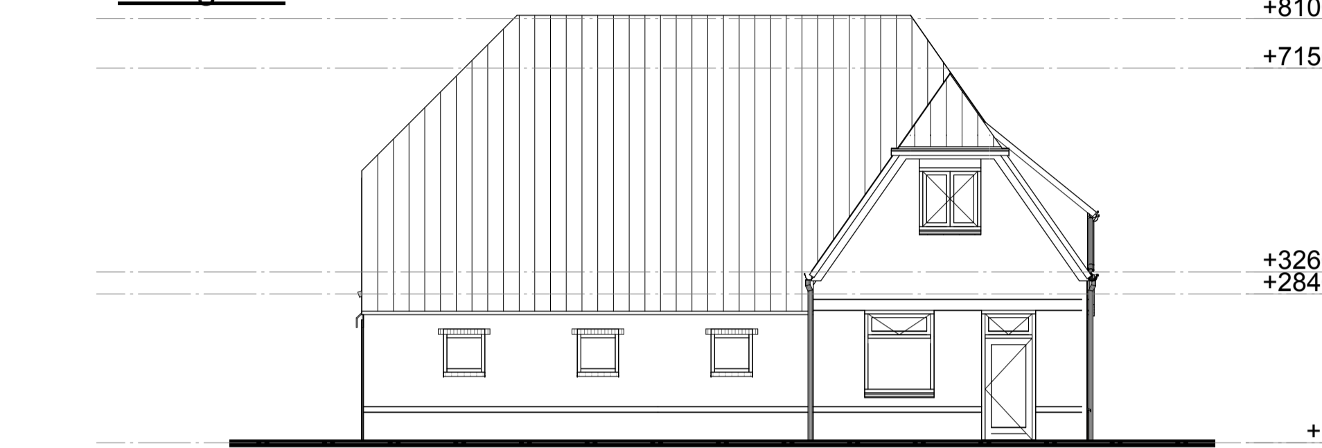
Linkergevel
