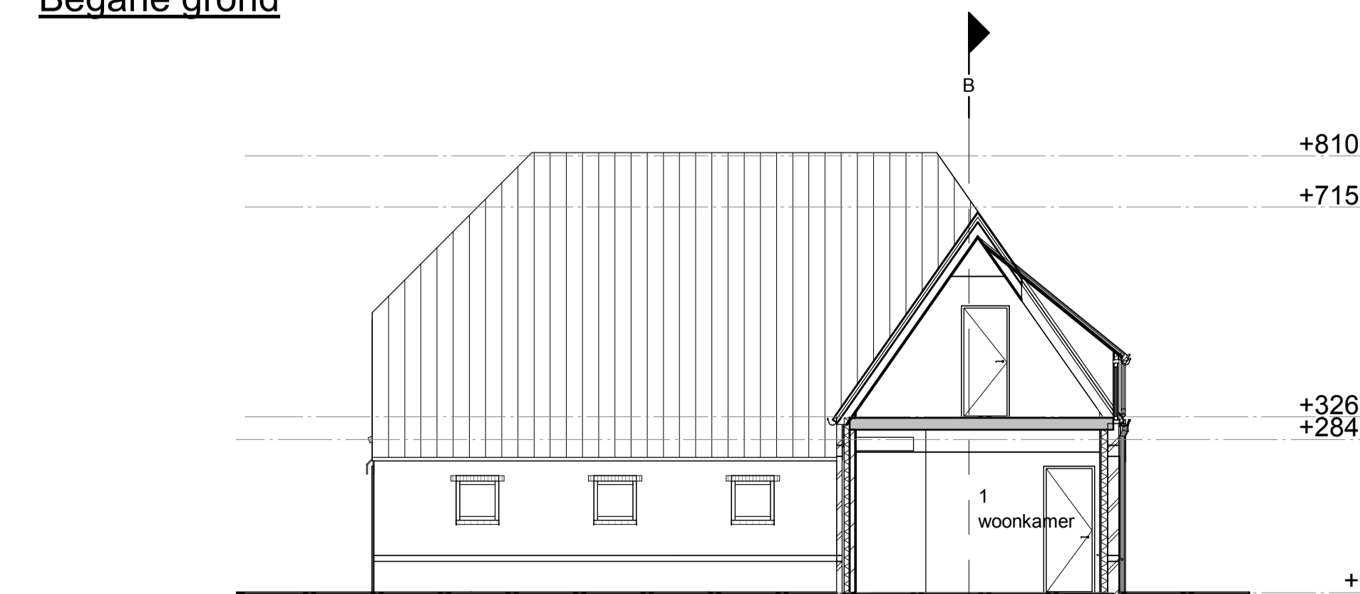
Doorsnede A
