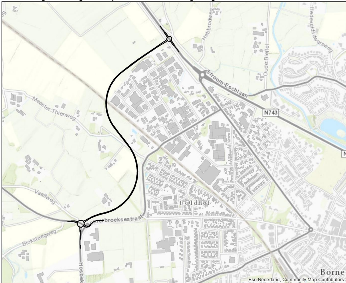
Afbeelding 3-1. Wegontwerp nieuwe verbindingsweg
