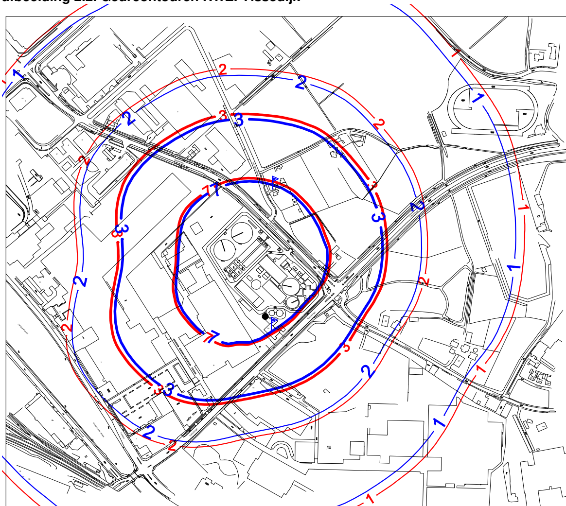
afbeelding 2.2. Geurcontouren RWZI Vissedijk 3
