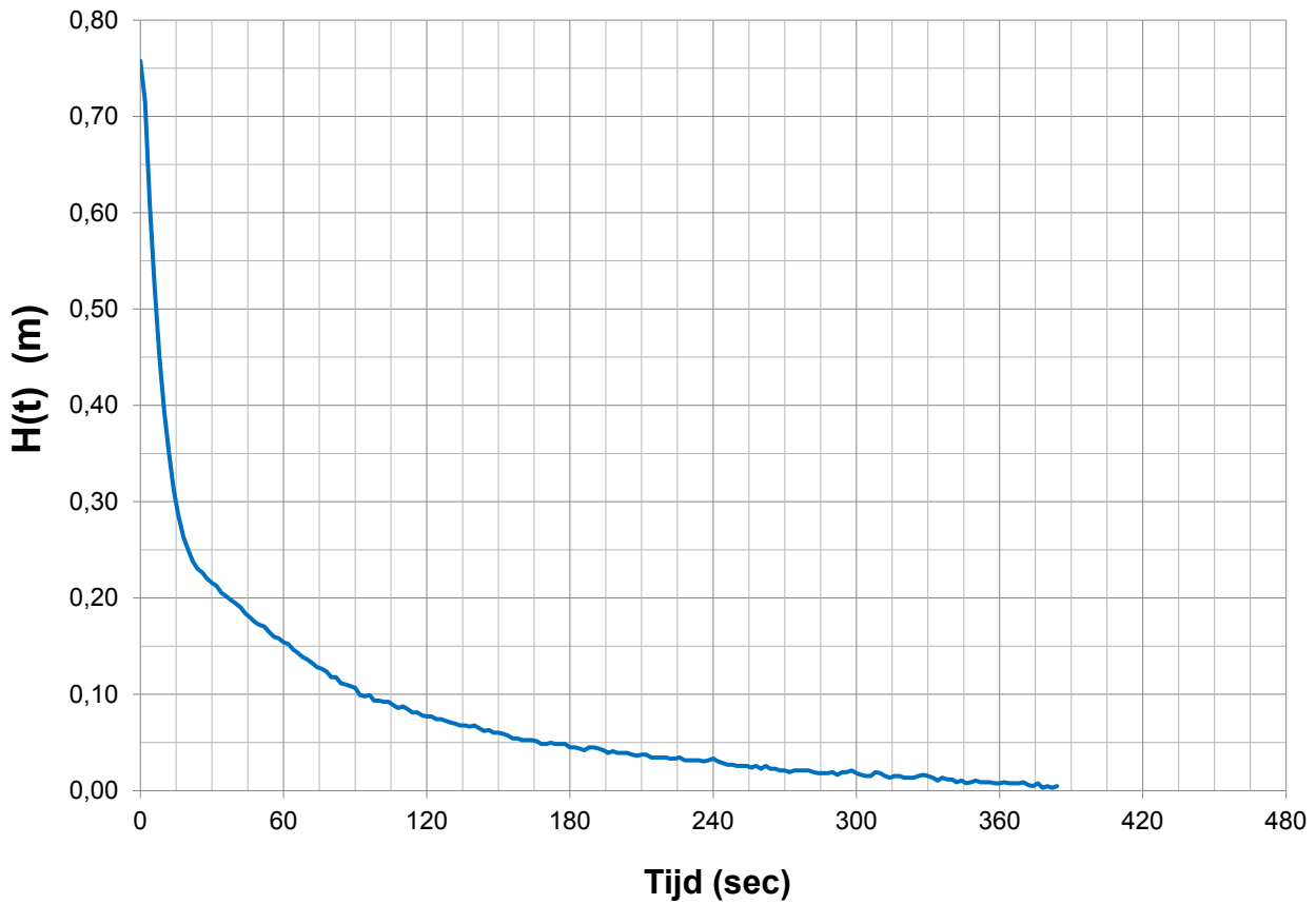
Heetveldsweg - Infiltratieproef H01 meting 1 : K = 1,8 m/dag
