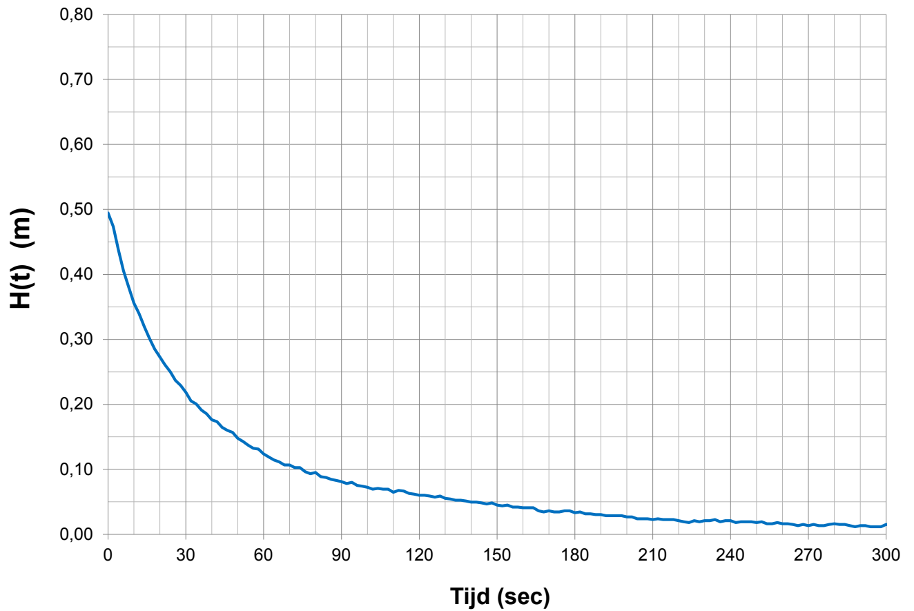
Heetveldsweg - Infiltratieproef H03 meting 2 : K = 1,1 m/dag
