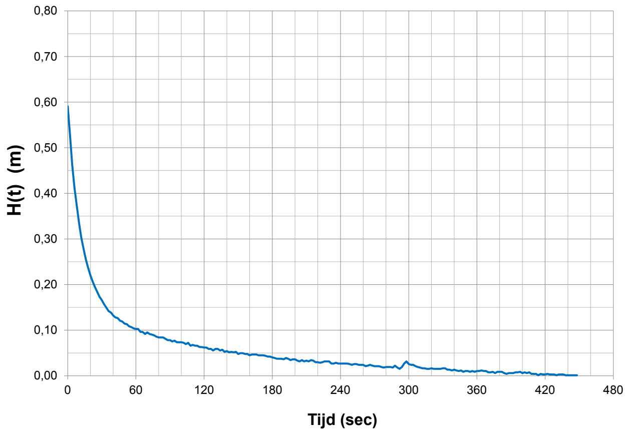
Heetveldsweg - Infiltratieproef H01 meting 2 : K = 1,9 m/dag
