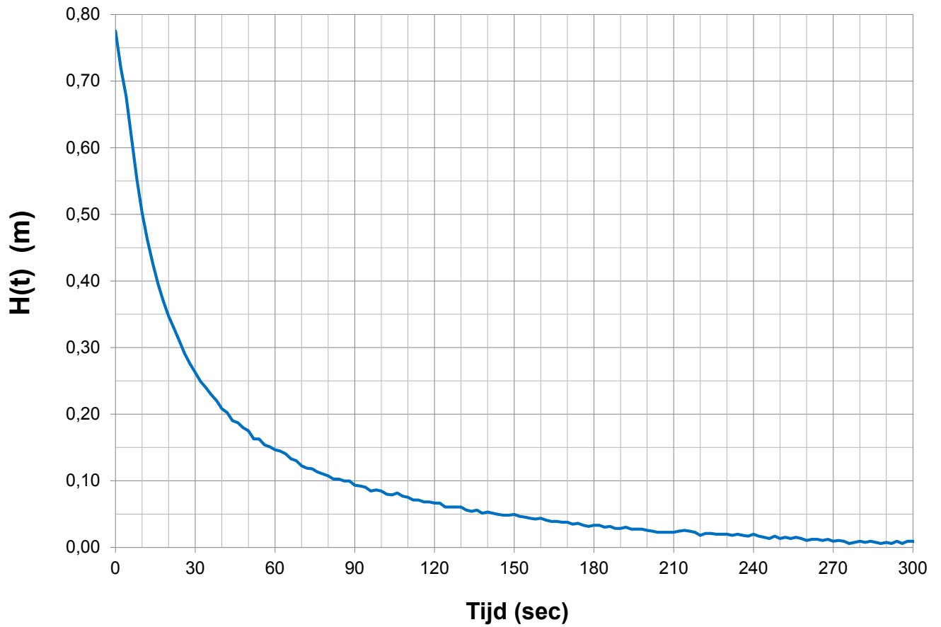
Heetveldsweg - Infiltratieproef H03 meting 1 : K = 1,4 m/dag
