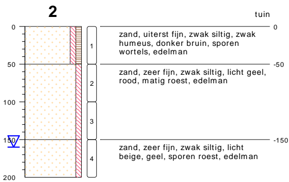
type grondboring datum 20-01-2017 boormeester Jan Hartman
