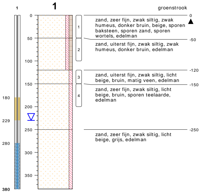
type peilbuis met 1 filter datum 20-01-2017 boormeester Jan Hartman
