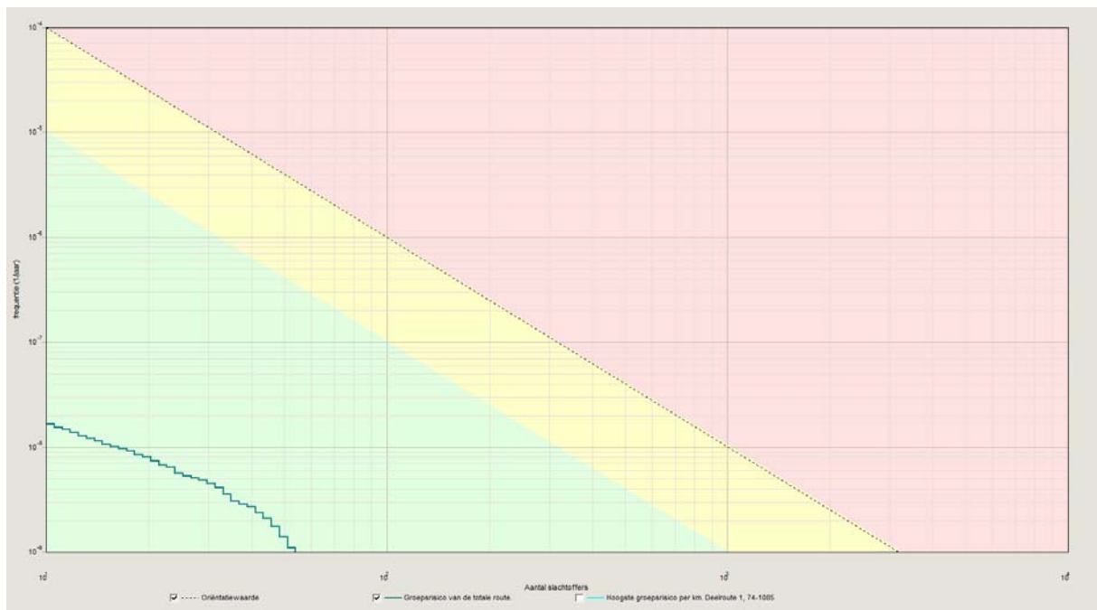
Afbeelding 4 f/N curve van het groepsrisico
