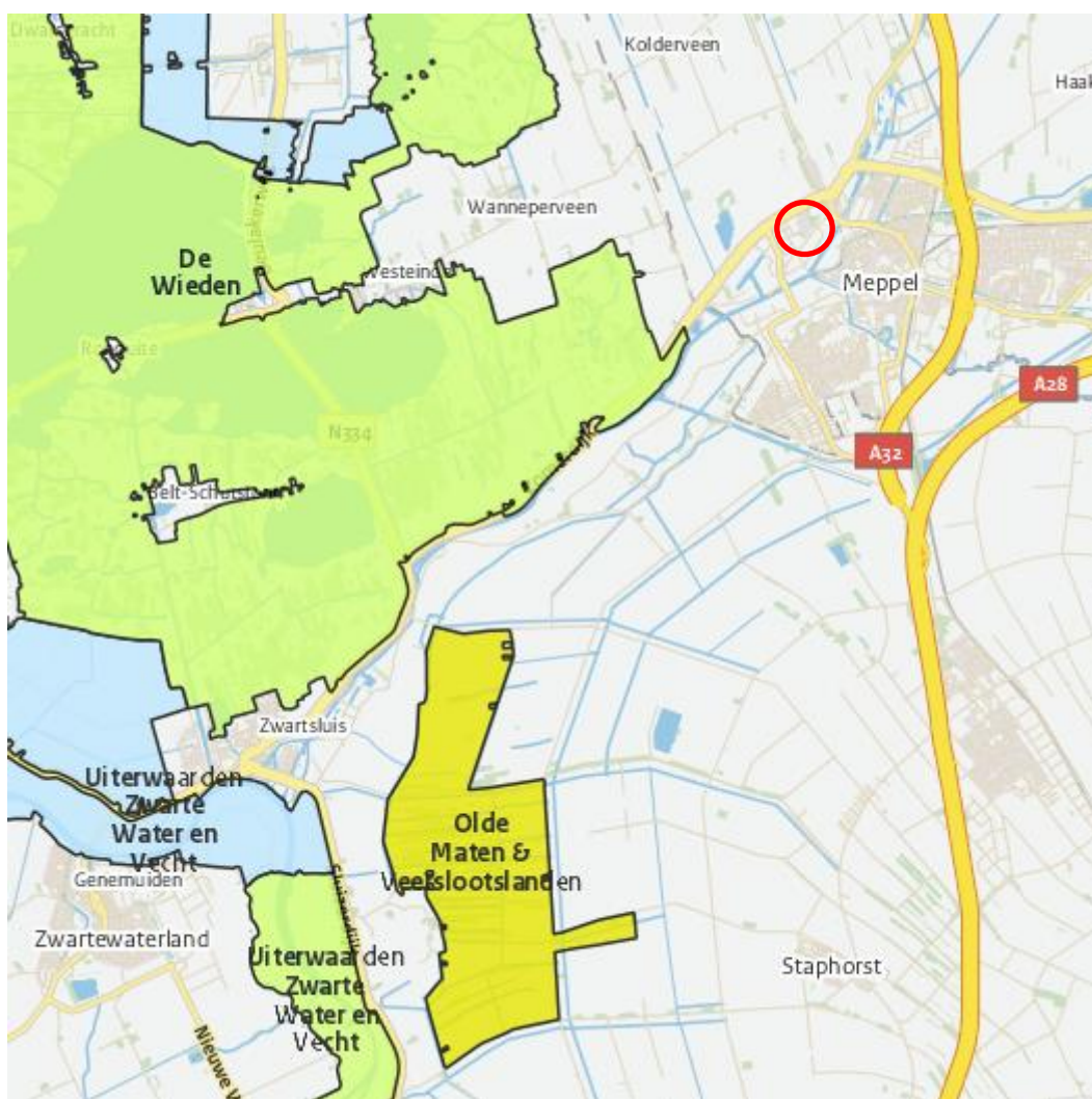
Figuur 1.1 Ligging plangebied t.o.v. Natura 2000-gebieden
