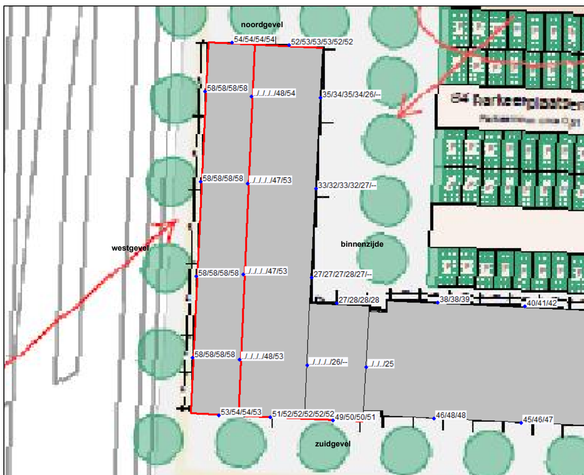
Figuur 4.1 Gevels met geluidbelasting > 48 dB
