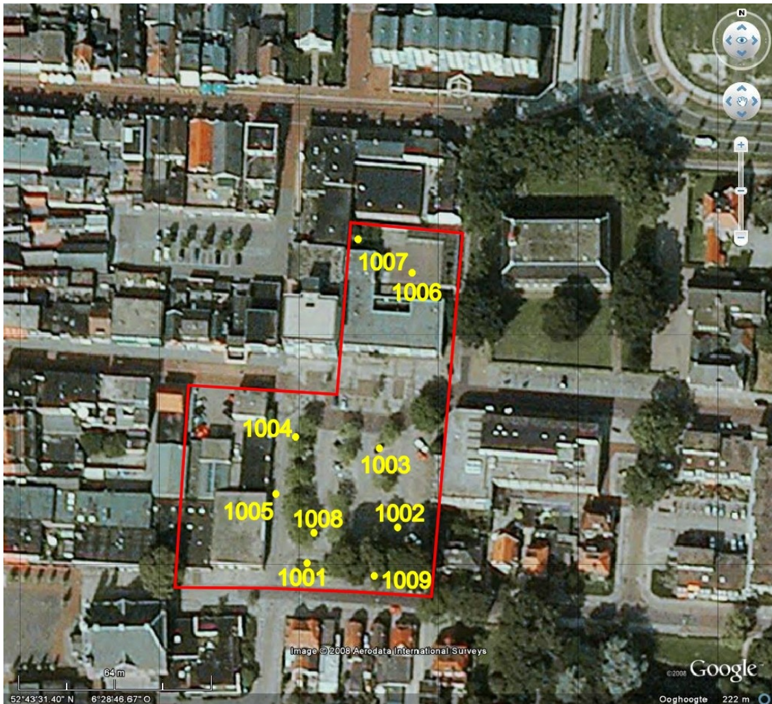
Figuur G: Hoogeveen, Bebouwde Kom: situatietekening van Locatie 10 Van Echtenplein met de boorlocaties. Met een rode lijn is de begrenzing van de onderzoekslocatie aangegeven. De genummerde punten geven de uitgevoerde boringen weer (RD-coördinaten NO – 228,832/527,054; ZO – 228,818/526,935; ZW – 228,738/526,941; NW – 228,796/527,055).
