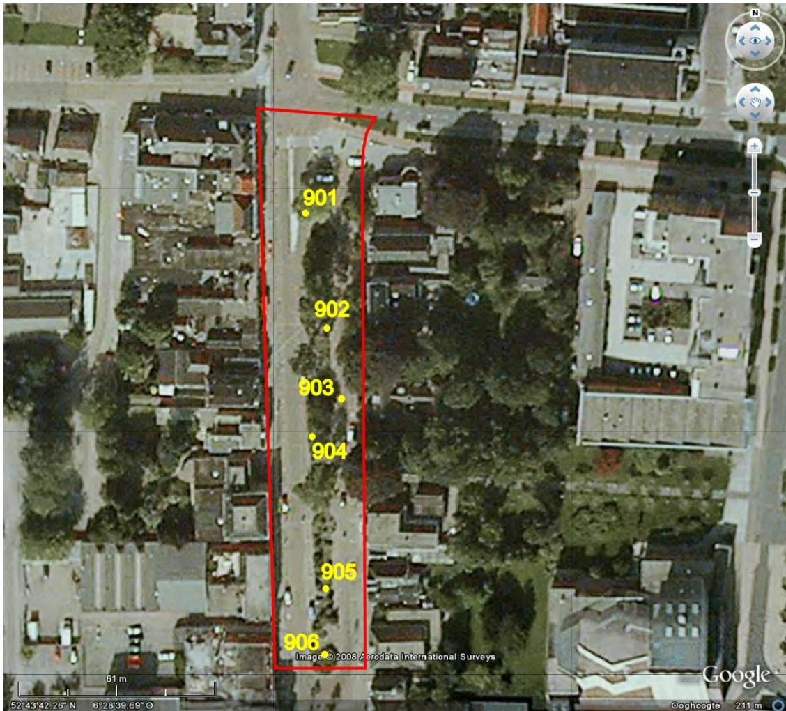
Figuur F: Hoogeveen, Bebouwde Kom: situatietekening van Locatie 9 Hoofdstraat Noord met de boorlocaties. Met een rode lijn is de begrenzing van de onderzoekslocatie aangegeven. De genummerde punten geven de uitgevoerde boringen weer (RD-coördinaten NO – 228,660/527,418; ZO – 228,663/527,244; ZW – 228,636/527,244; NW – 228,627/527,421).
