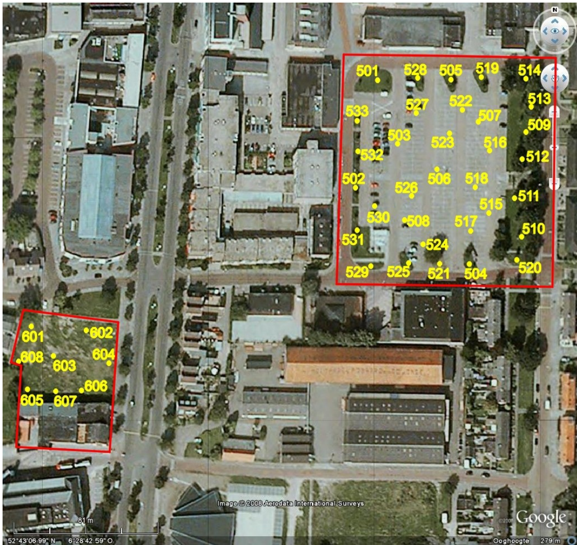
Figuur D: Hoogeveen, Bebouwde Kom: situatietekening van Locatie 5 Beukema-plein en Locatie 6 Alteveer met de boorlocaties. Met een rode lijn zijn de begrenzingen van de onderzoekslocaties aangegeven. De genummerde punten geven de uitgevoerde boringen weer (RD-coördinaten Locatie 5 Beukema-plein NO – 228,891/526,371; ZO – 228,890/526,247; ZW – 228,767/526,248; NW – 228,770/526,371; Locatie 6 Alteveer NO – 228,652/526,627; ZO – 228,649/526,155; ZW – 228,595/526,155; NW – 228,596/526,234).
