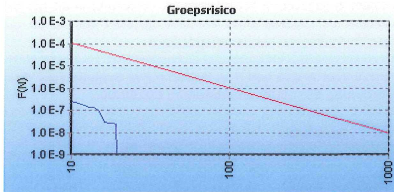
5.4 Figuur 5.7 FN curve voor A-661 van N.V. Nederlandse Gasunie voor de kilometer tussen stationing 59640.00 en stationing 60640.00
