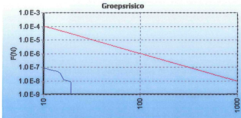
5.2 Figuur 5.5 FN curve voor A-519 van N.V. Nederlandse Gasunie voor de kilometer tussen stationing 71470.00 en stationing 72470.00
