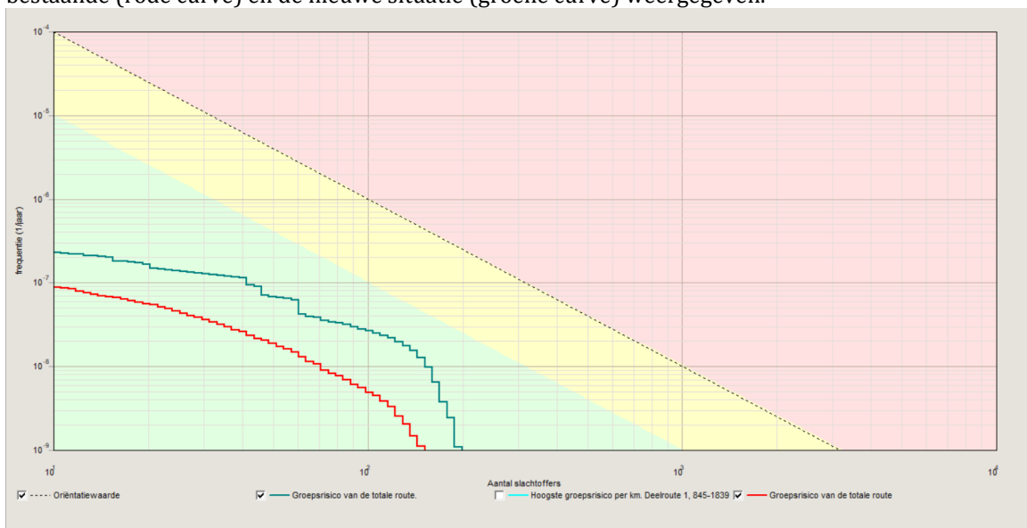
Figuur 6. Groepsrisicocurve
