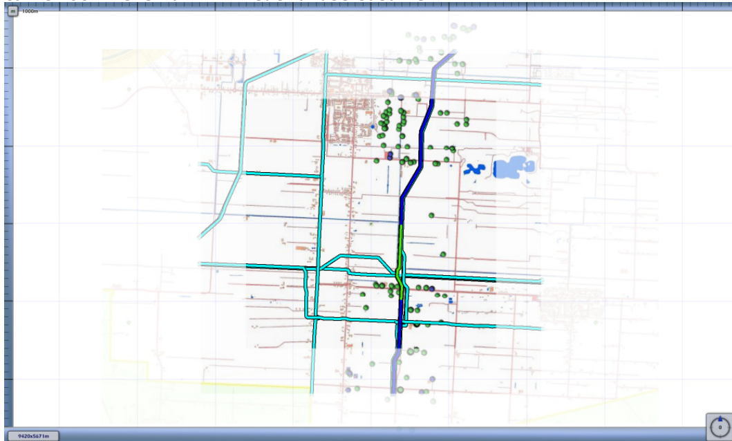
Figuur 4.4 Kilometer leiding behorende bij de maximale overschrijding van de FN-curve voor A-519 van N.V. Nederlandse Gasunie
