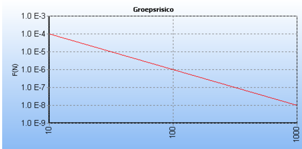
5.6 Figuur 5.16 FN curve voor N-525-40 van N.V. Nederlandse Gasunie voor de kilometer tussen stationing 7940.00 en stationing 8940.00
