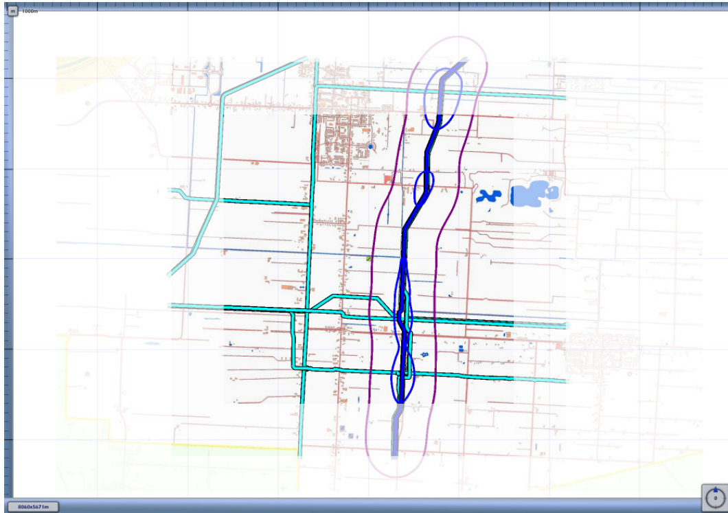
3.2 Figuur 3.4 Plaatsgebonden risico voor A-519 van N.V. Nederlandse Gasunie
