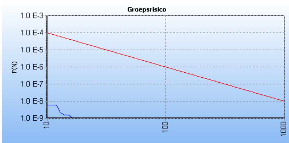
5.2 Figuur 5.4 FN curve voor A-519 van N.V. Nederlandse Gasunie voor de kilometer tussen stationing 76180.00 en stationing 77180.00
