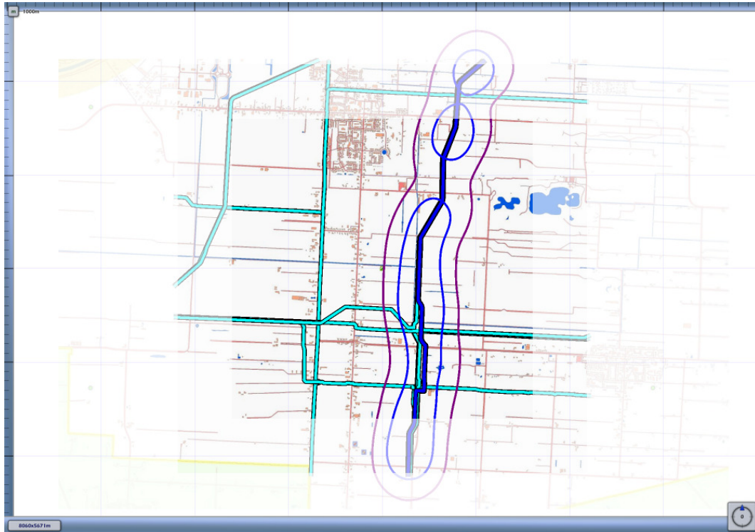
3.5 Figuur 3.12 Plaatsgebonden risico voor A-661 van N.V. Nederlandse Gasunie
