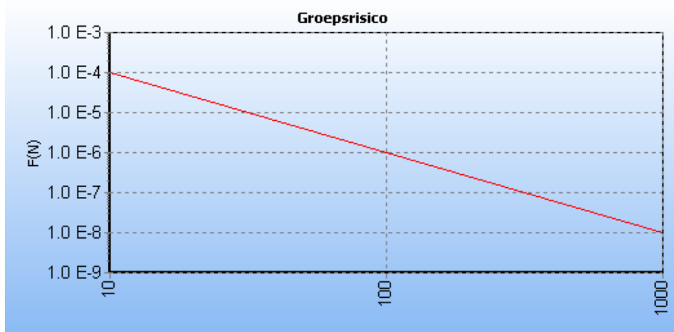
5.5 Figuur 5.12 FN curve voor A-661 van N.V. Nederlandse Gasunie voor de kilometer tussen stationing 64240.00 en stationing 65240.00
