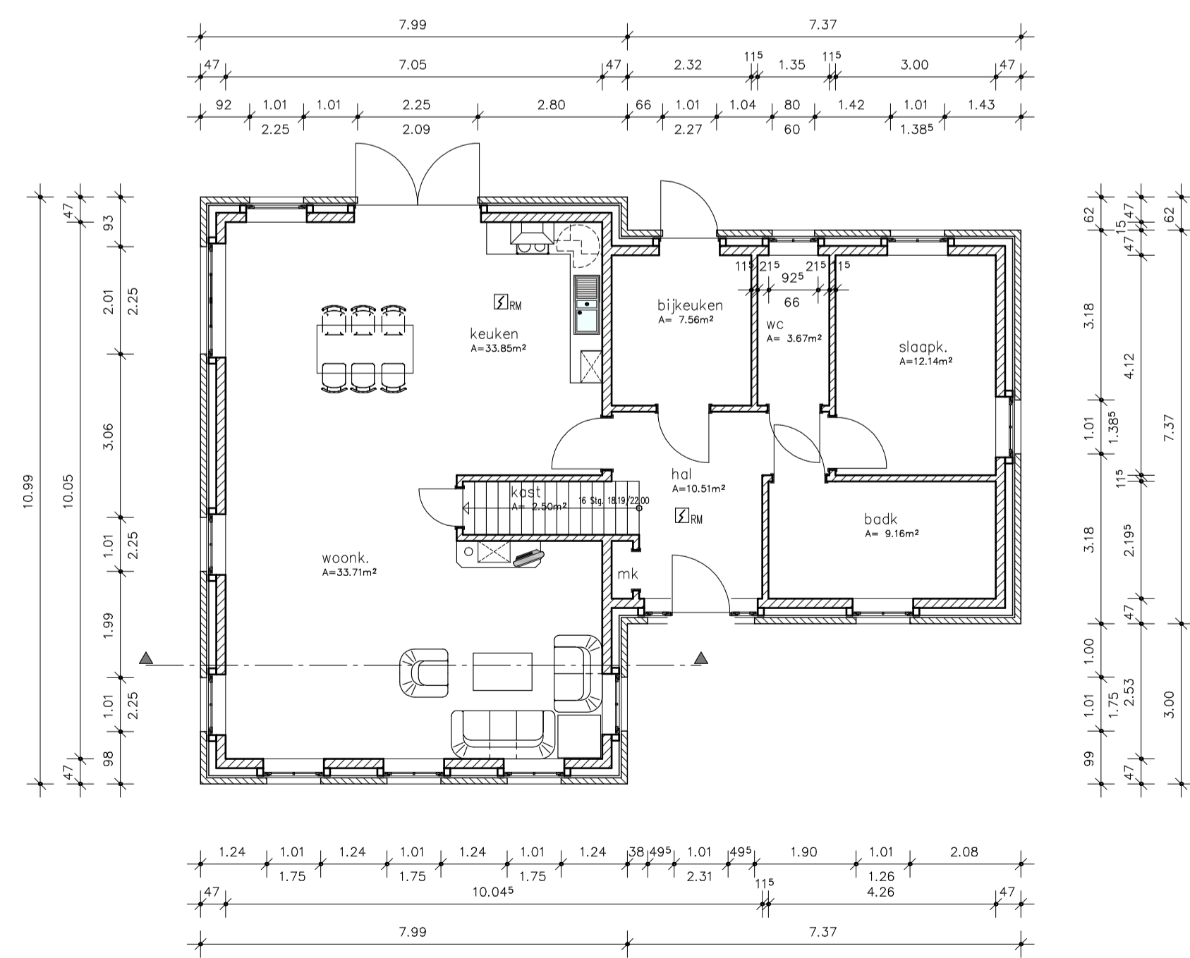
Begane Grond
