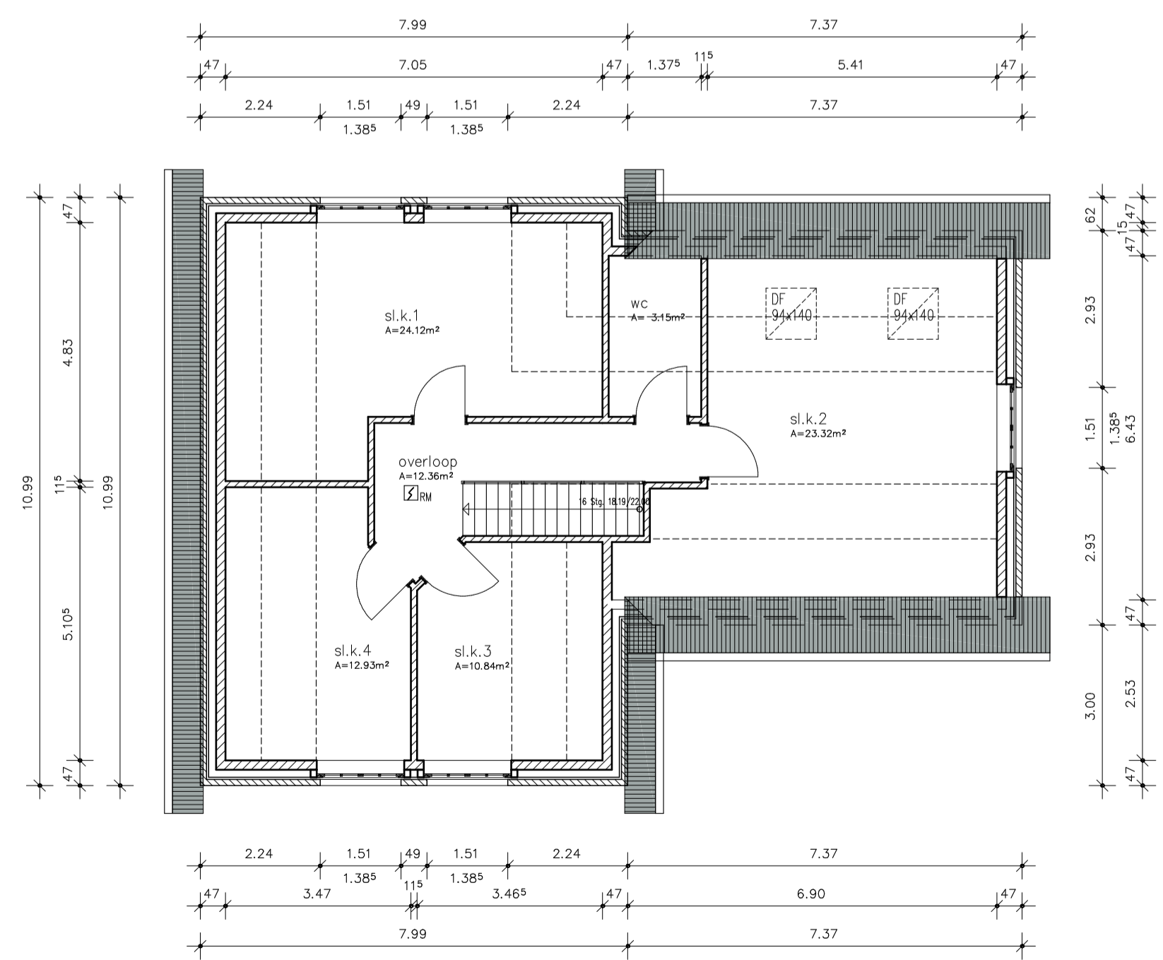
Verdieping
