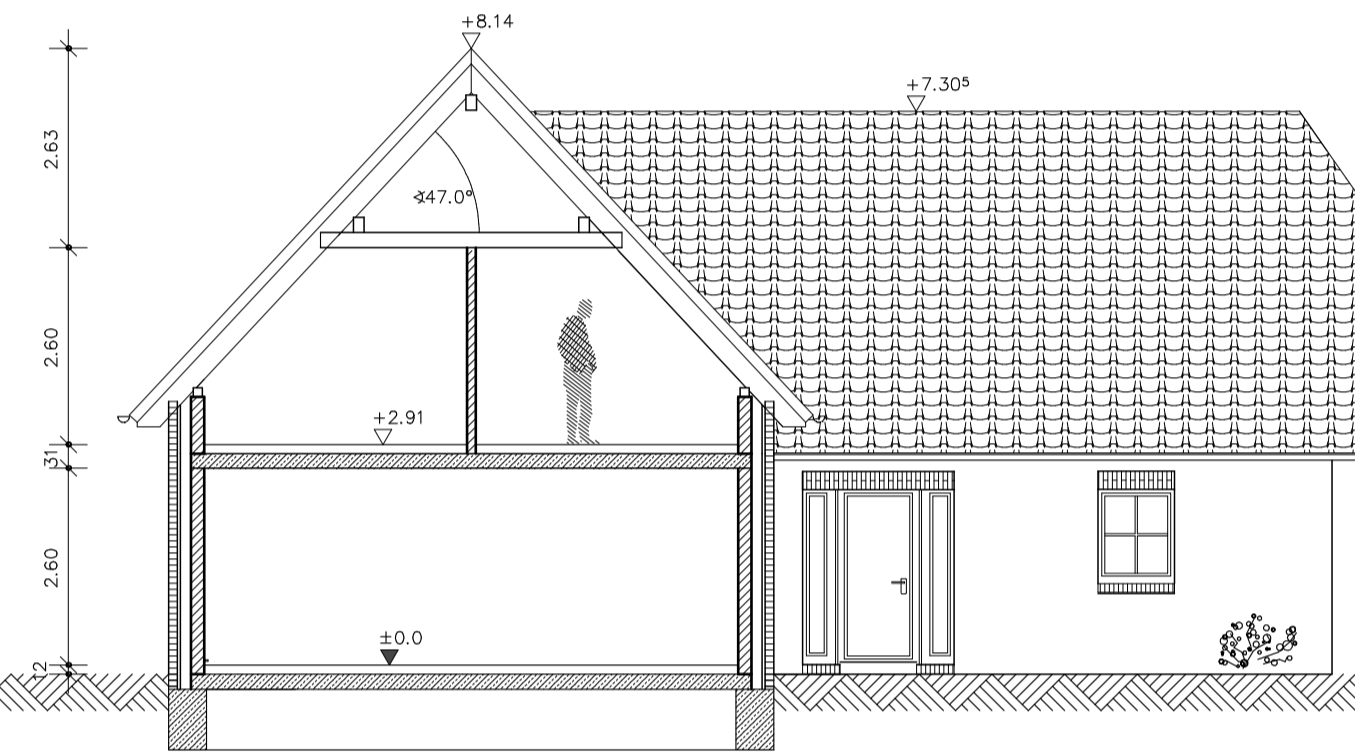
Doorsnede
