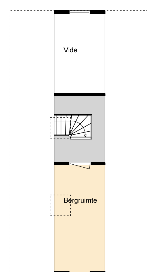
Verdieping bijgebouw
