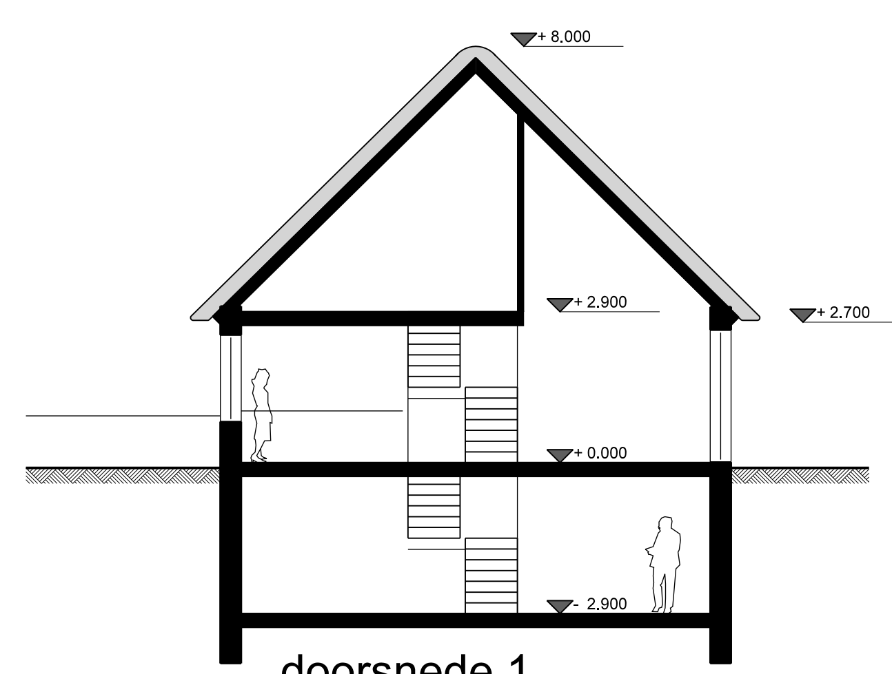
doorsnede 1
