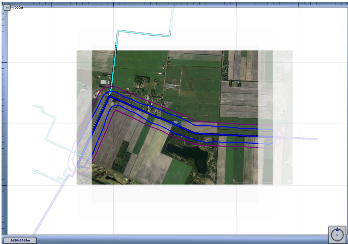
3.1 Figuur 3.2 Plaatsgebonden risico voor 5072_leiding-A-582-deel-1 van N.V. Nederlandse Gasunie
