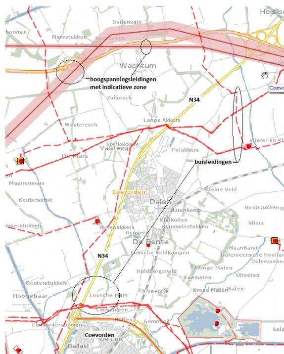
Figuur 4.1: overzicht kruisende buisleidingen en hoogspanningsleidingen met de N34
