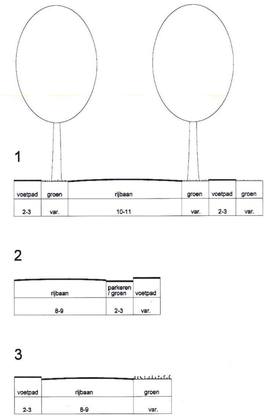
dwarsprofielen schaal 1 : 200
