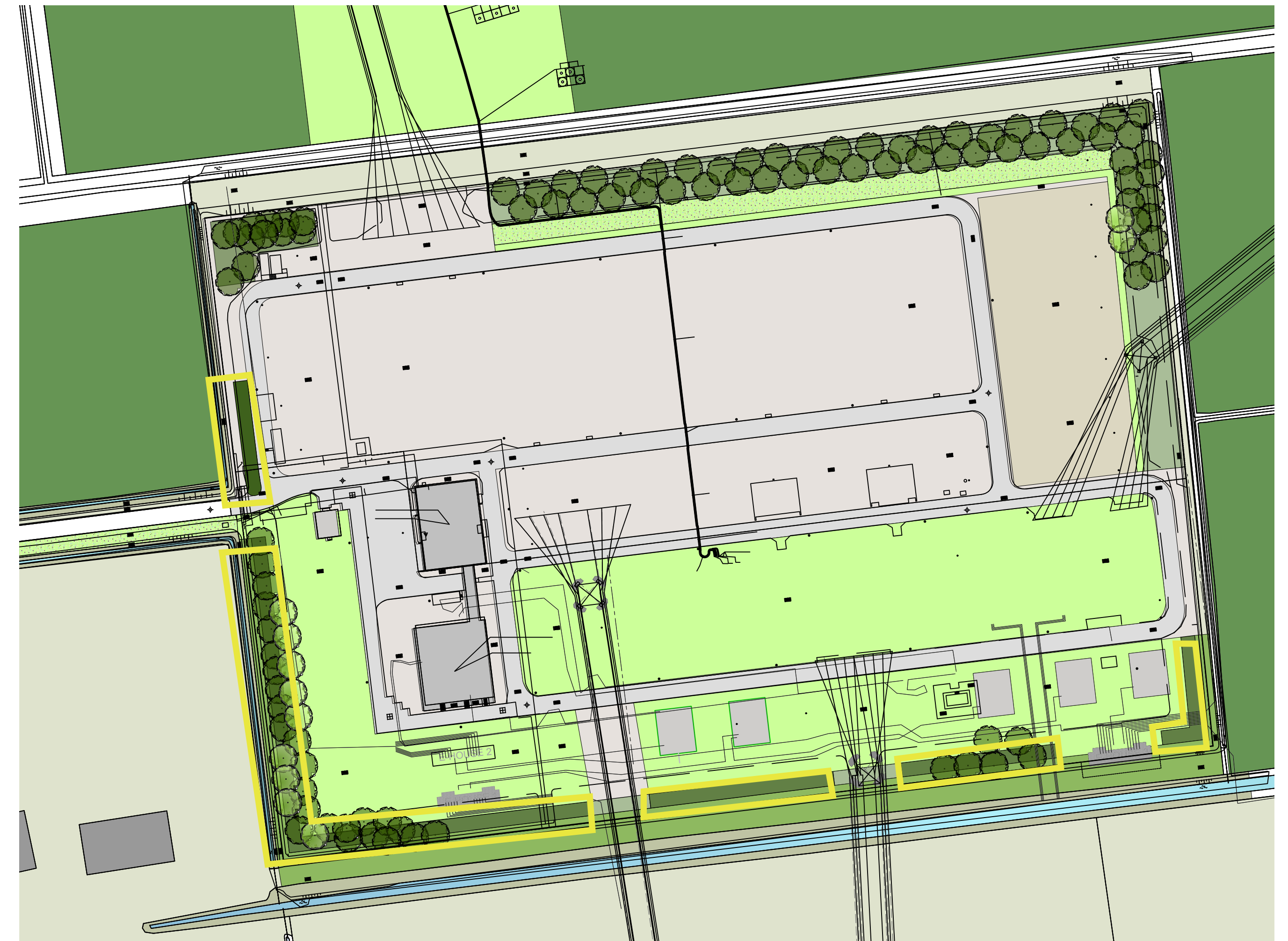
Locaties hoog struweel Ontwerp plattegrond schaal 1:1000
