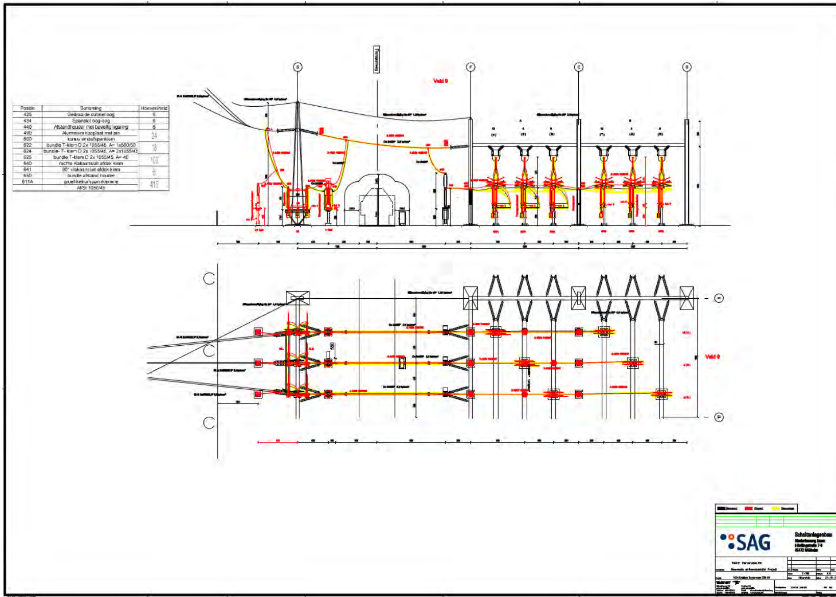
Bijlage C-6 Tekening zijaanzicht 220kV lijnveld 9
