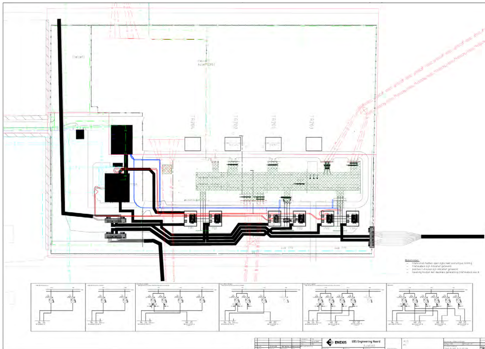
Bijlage C-17 Tekening bovenaanzicht uitbreidingen Enexis met locaties E-houses en tracés 20kV- en 10kV-transformatorkabels
