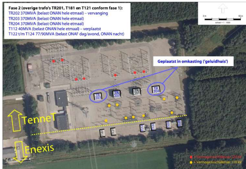
Figuur 5.2 Globale lay-out (alleen relevante geluidbronnen) na uitbreiding/wijziging fase 2
