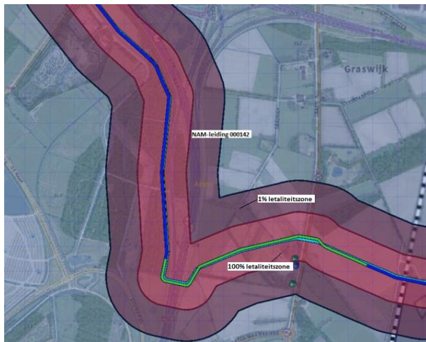
Figuur 10: Ligging 1%- en 100% letaliteitszone buisleiding 000142 (bestaande situatie)
