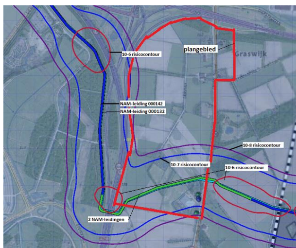
Figuur 9: Ligging plangebied met de 2 NAM-leidingen
