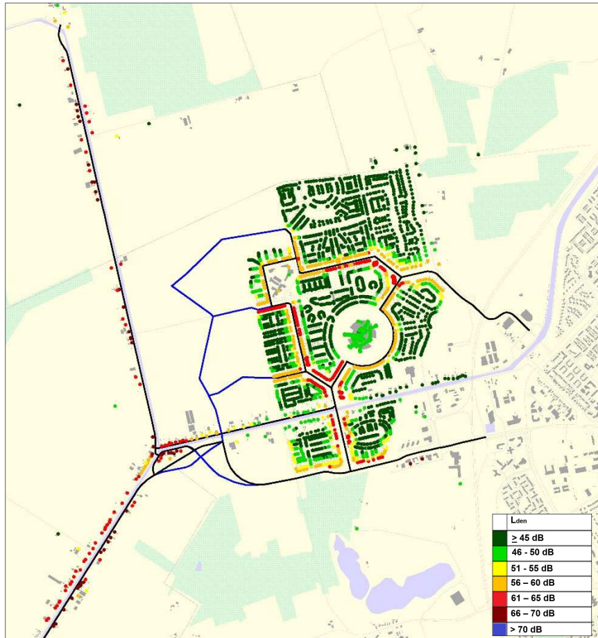
Figuur 5.5: Absolute geluidsbelastingen alternatief verspreid (cumulatief)
