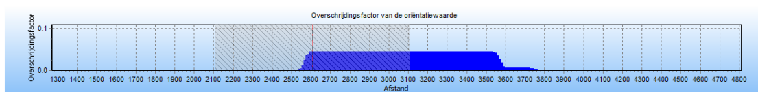
Figuur 5.5: Overschrijdingsfactor v/h GR over de hele berekende leiding (nieuwe situatie)
