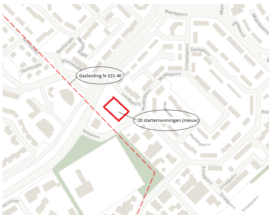
Figuur 4.2 : Overzicht van bebouwing rondom de Gasunieleiding N-521-40 (rode stippellijn)
