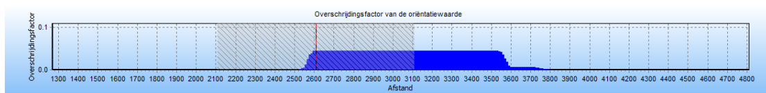
Figuur 5.3: Overschrijdingsfactor v/h GR over de hele berekende leiding (bestaande situatie)
