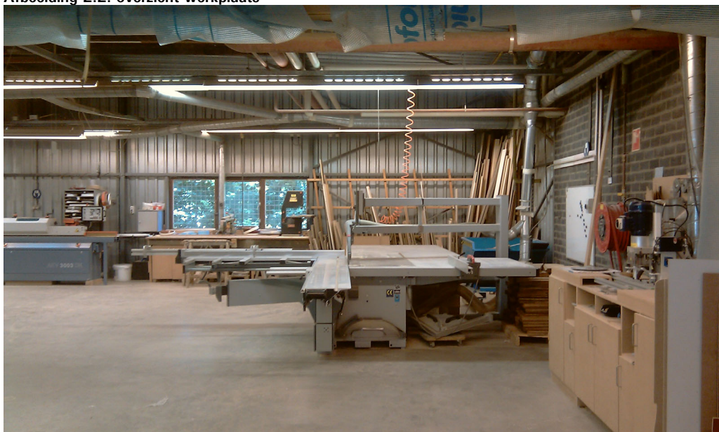
Afbeelding 2.2: overzicht werkplaats
