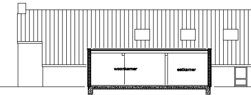
LANGS DOORSNEDE
