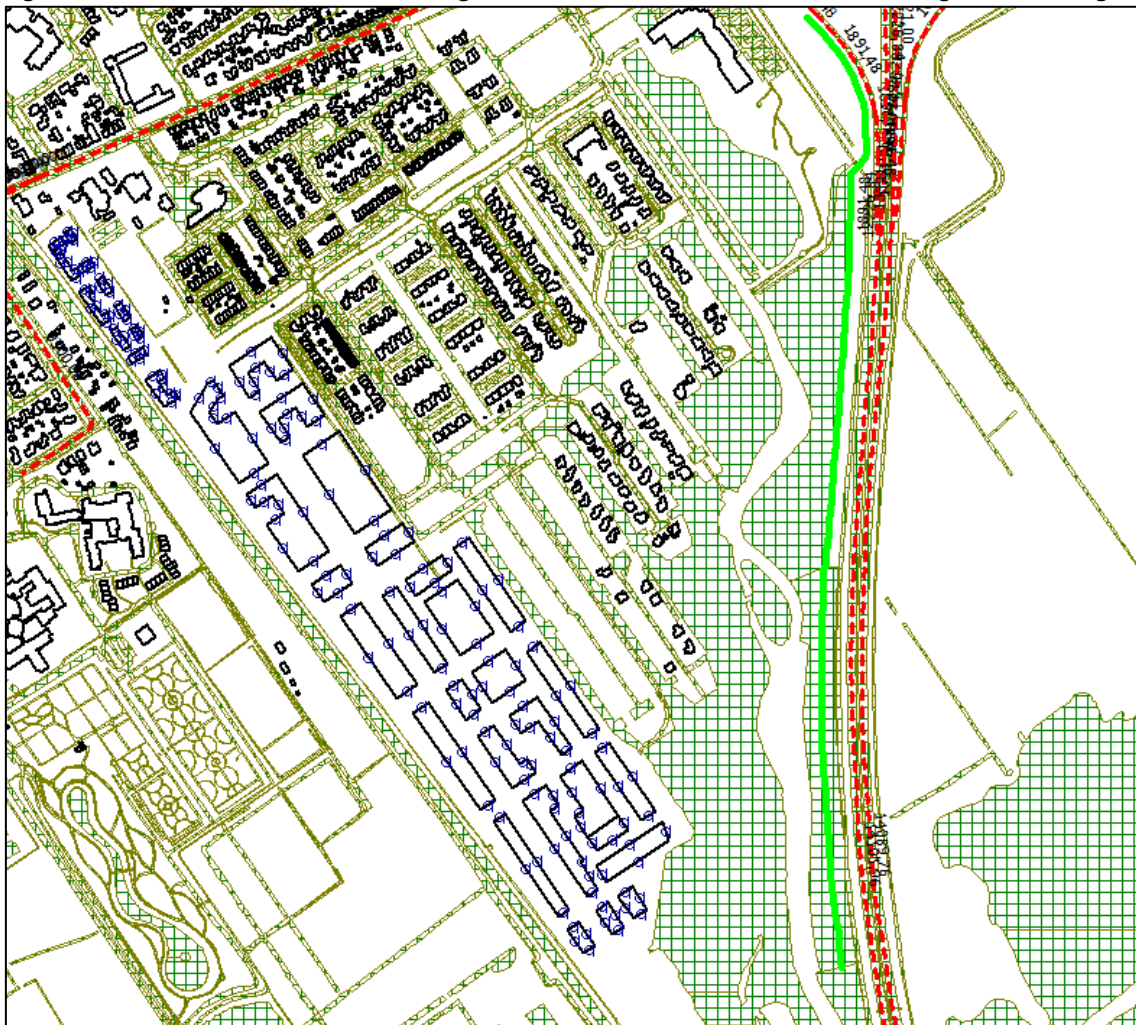
Figuur 4.1: overzicht van het wegverkeerslawaai rekenmodel met de ingevoerde wegen
