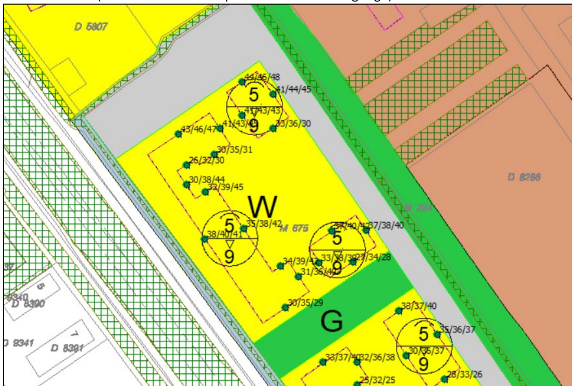
Figuur 5.1: overzicht van de berekende geluidbelasting L_{den} in dB vanwege de Lycklamaweg (inclusief 5 dB aftrek op basis van artikel 110g Wgh)
