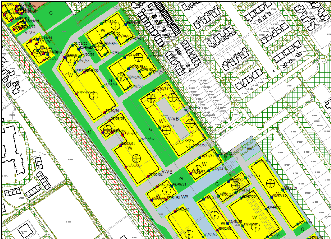
Figuur 5.5: overzicht van de berekende geluidbelasting L_{den} in dB vanwege de spoorlijn Leeuwarden-Zwolle
