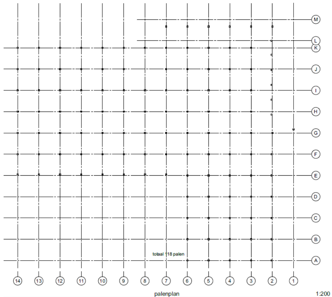
Figuur 2.8 Palenplan
