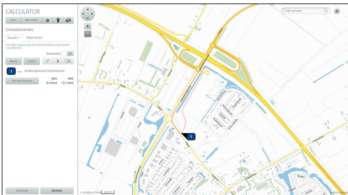
Afbeelding 3 - AERIUS model
