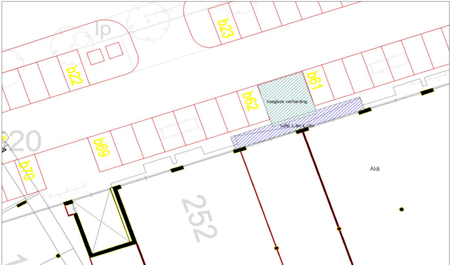
Principe beperking geluidsbelasting op gevels van de bovenliggende woningen ter plaatse van de entree van een supermarkt in de noordgevel van het winkelcentrum Noorderpoort
