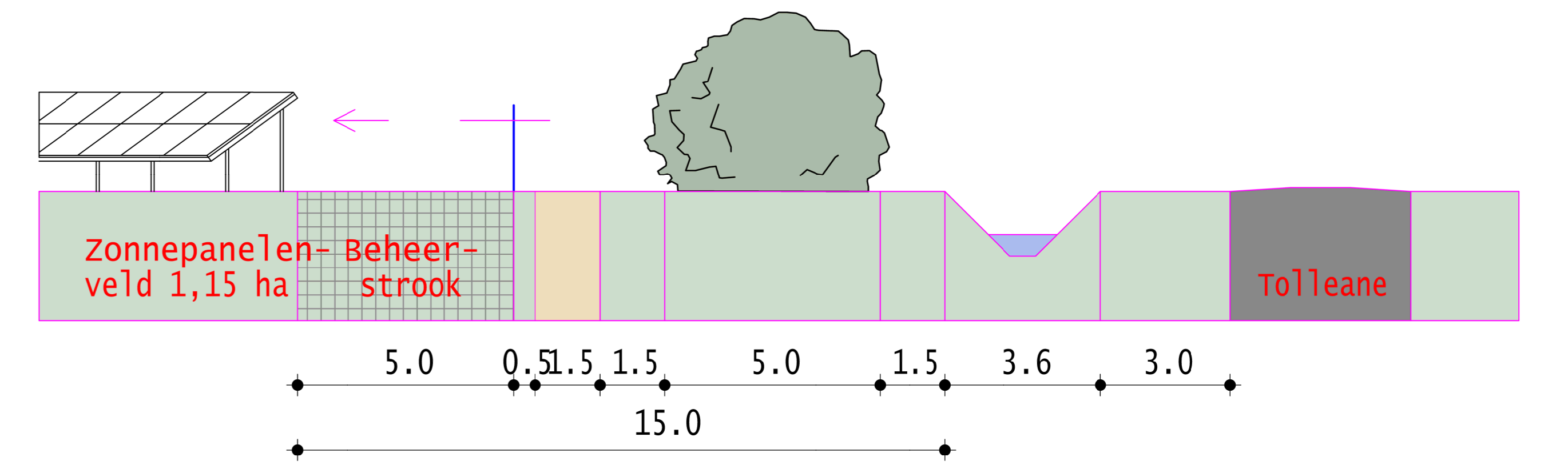
PROFIEL 2. ZUIDOOSTRAND - TOLLEANE
