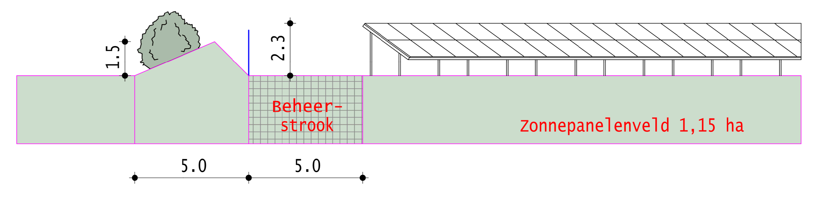
PROFIEL 1. NOORDWESTSTRAND
