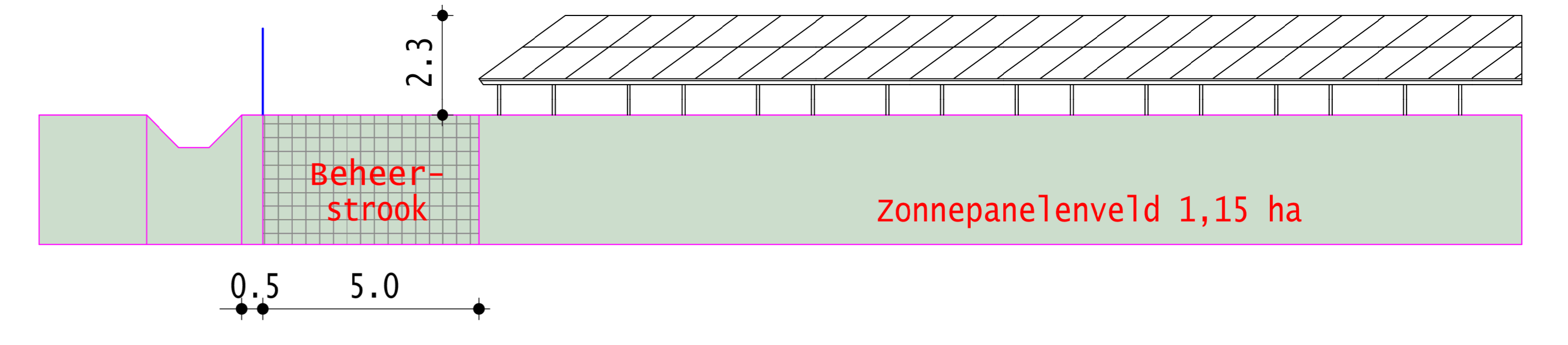
PROFIEL 3. ZUIDOOSTRAND
