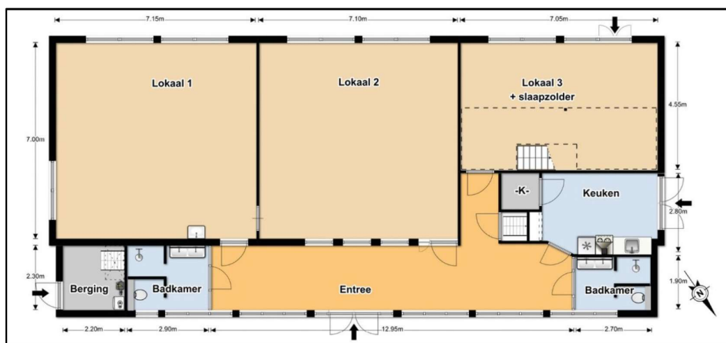
Figuur 4: Plattegrond/indeling voormalig schoolgebouw Ulesprong 18 Tijnje
