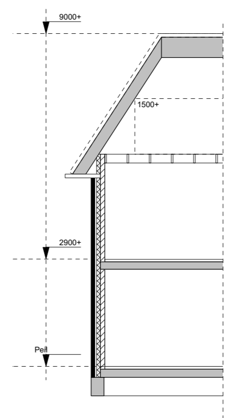
DOORSNEDE
