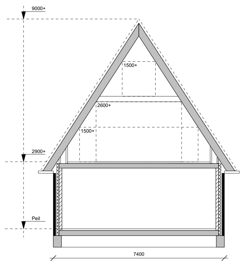
DOORSNEDE
