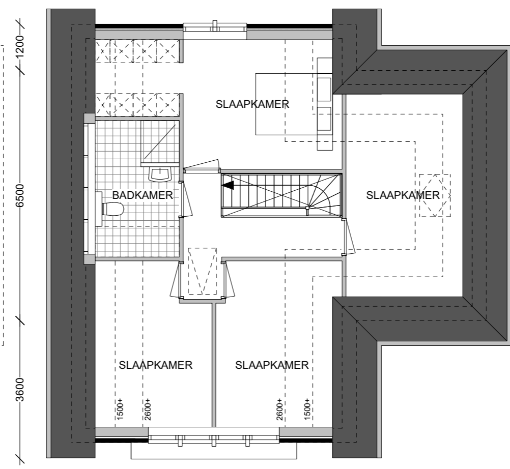
VERDIEPING
