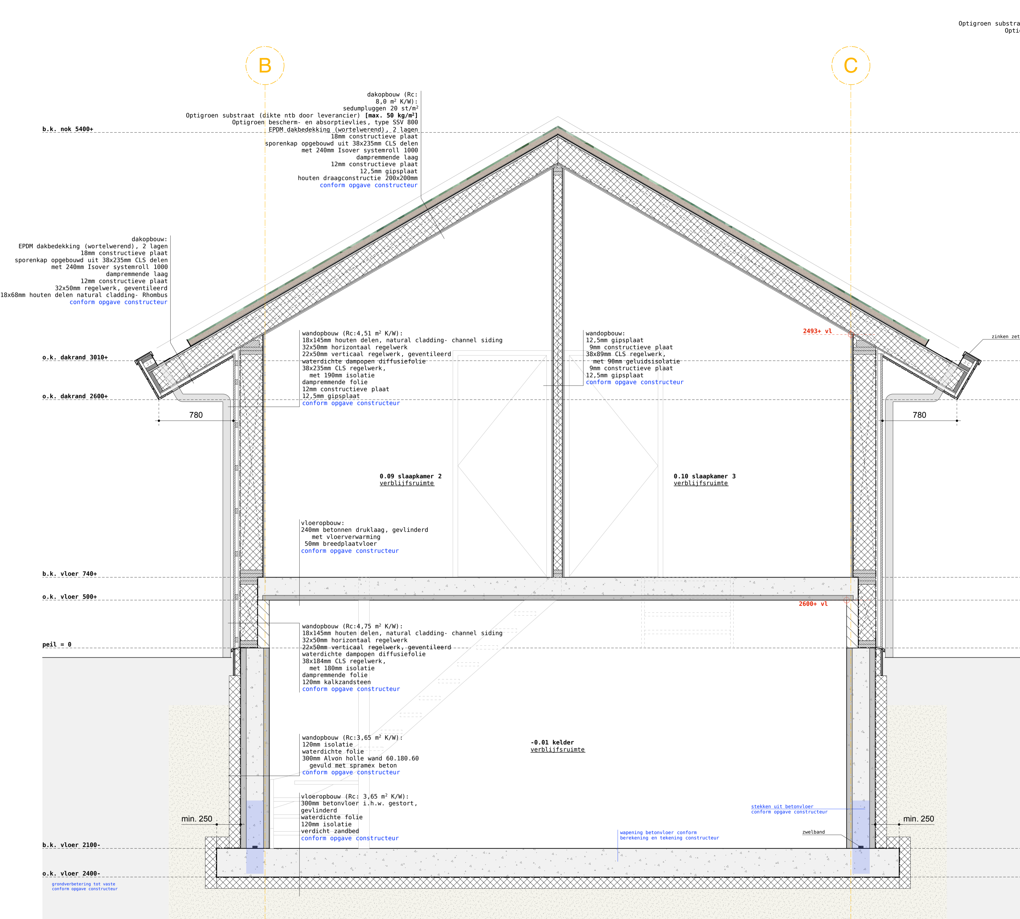
doorsnede a
