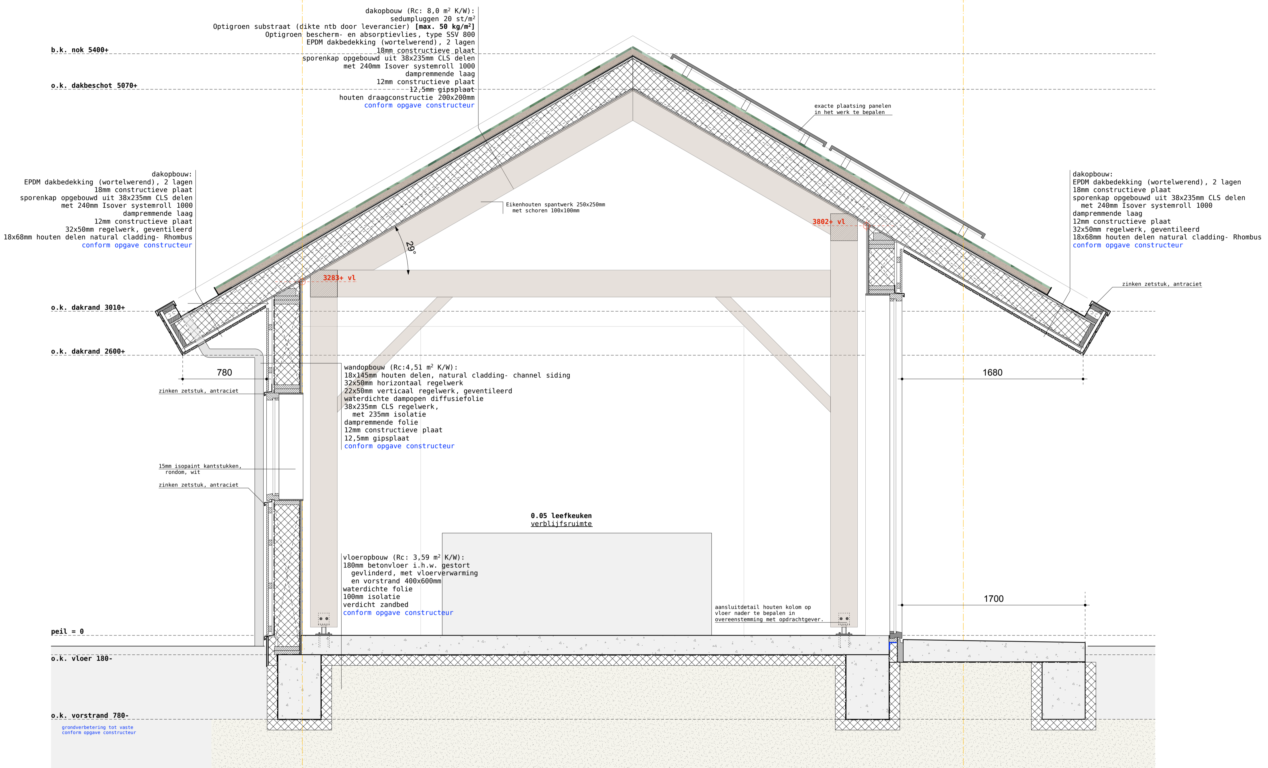
doorsnede c
