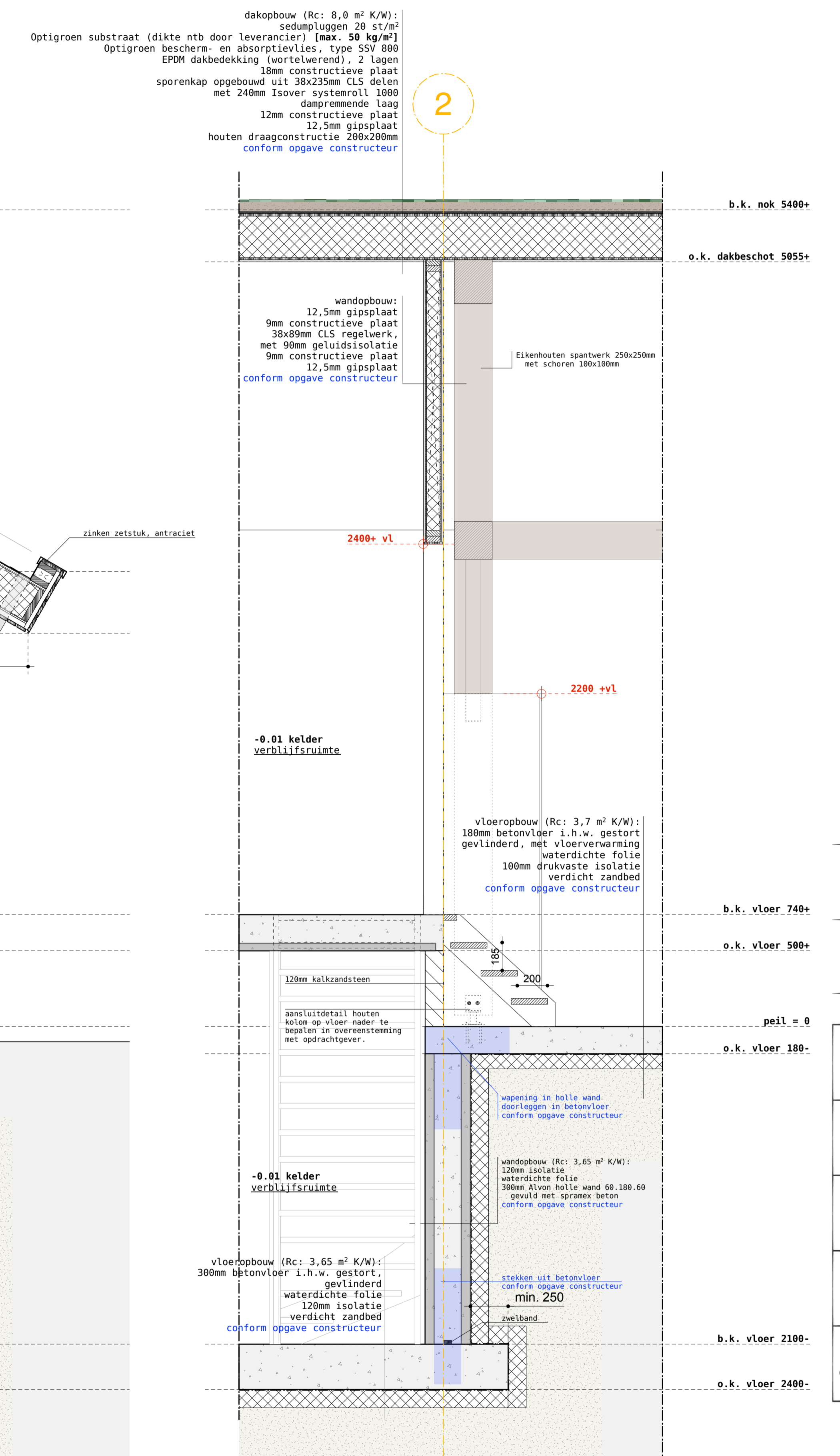
doorsnede f
