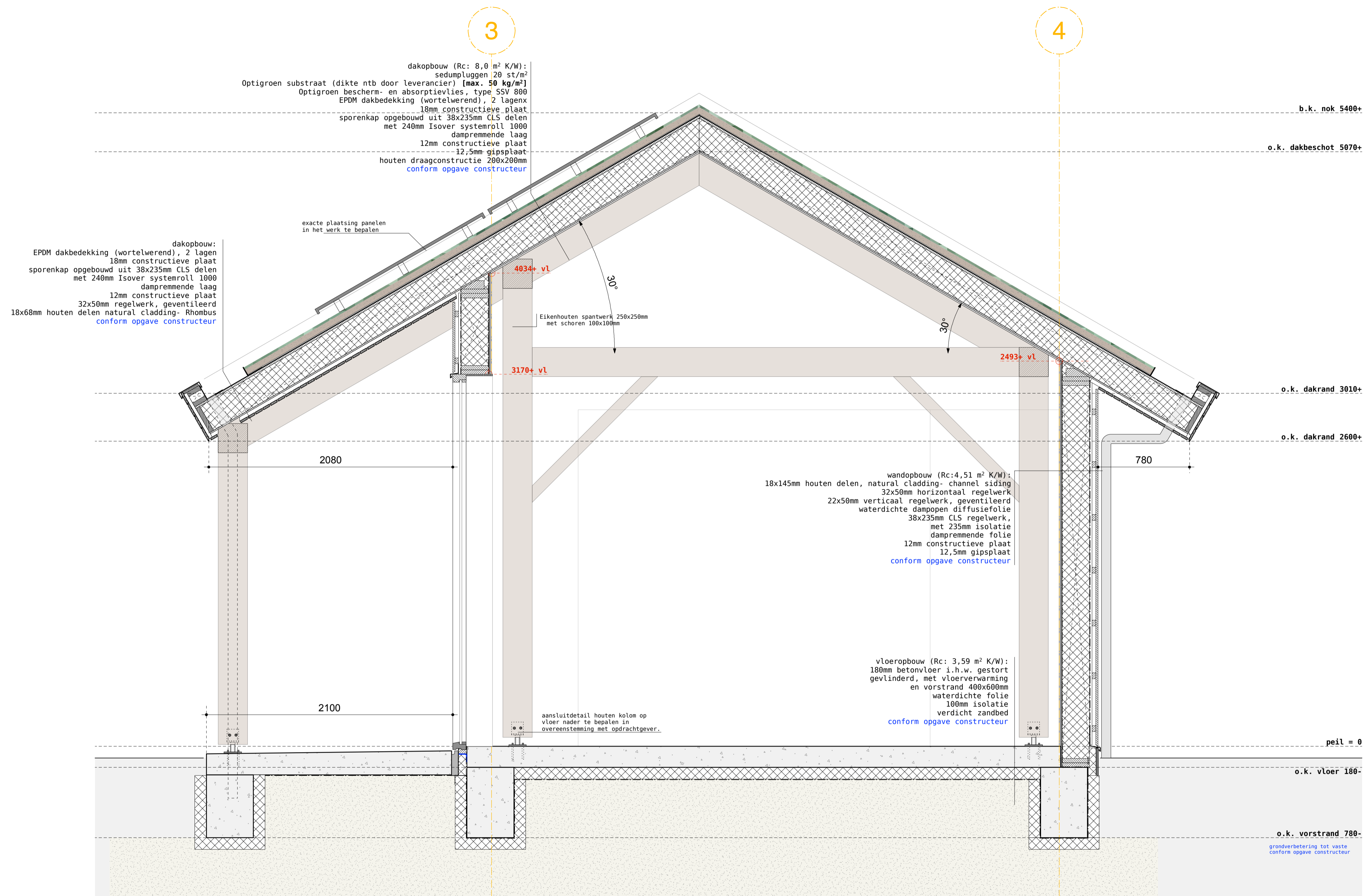
doorsnede d
