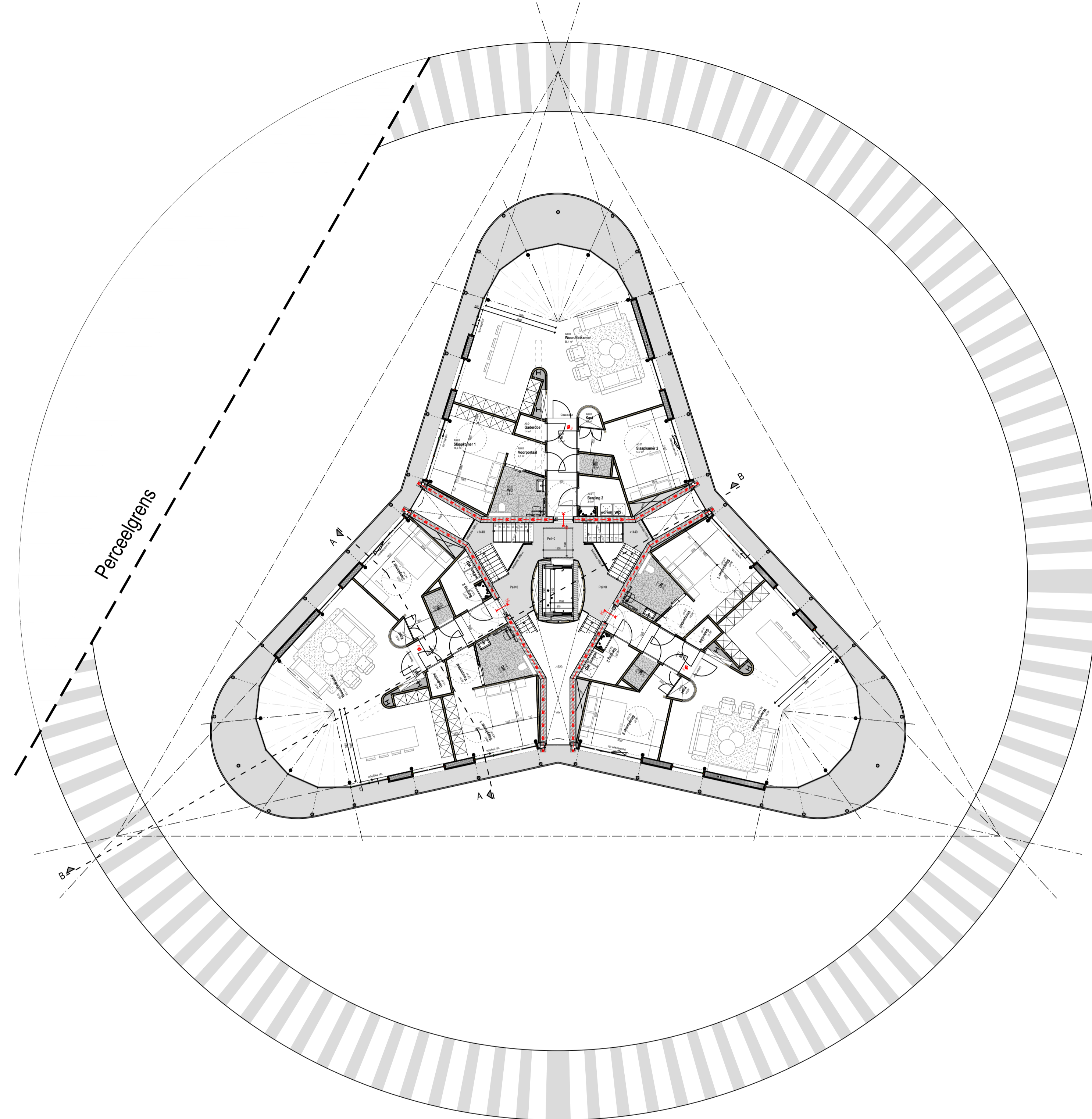
1e VERDIEPING
