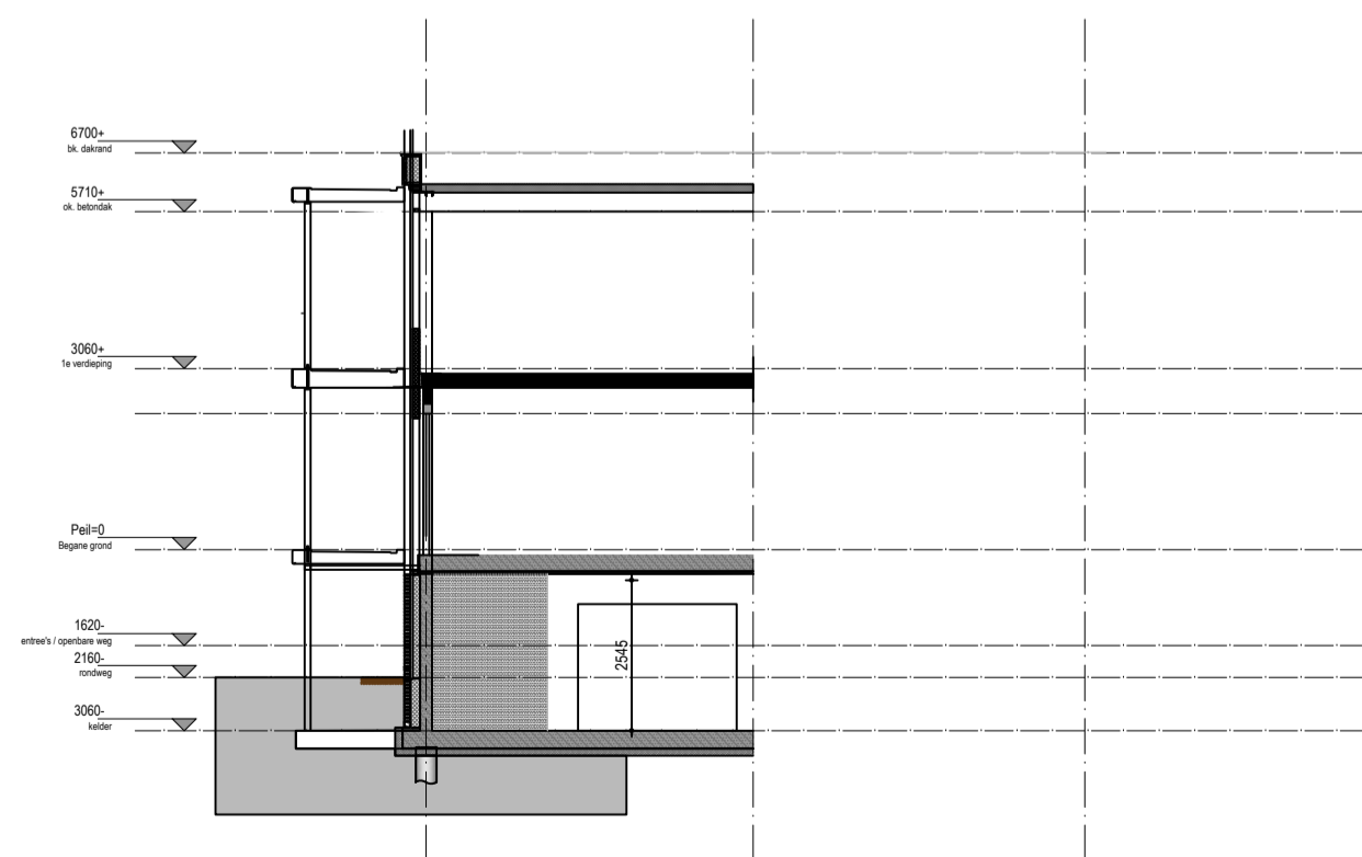
DOORSNEDE A-A
