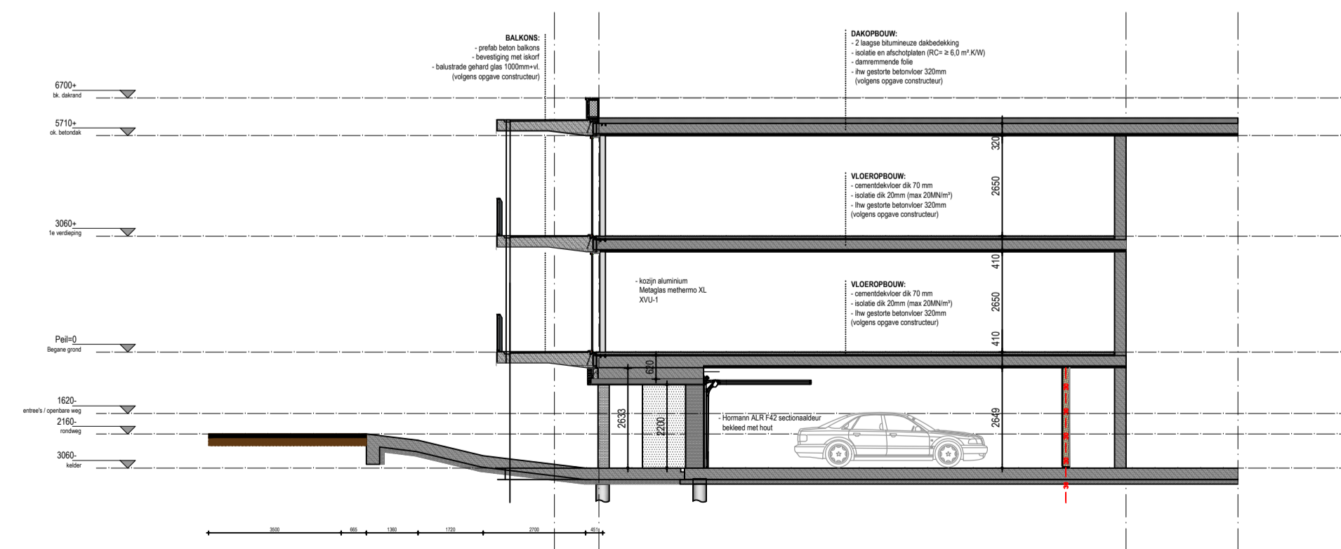
DOORSNEDE B-B
