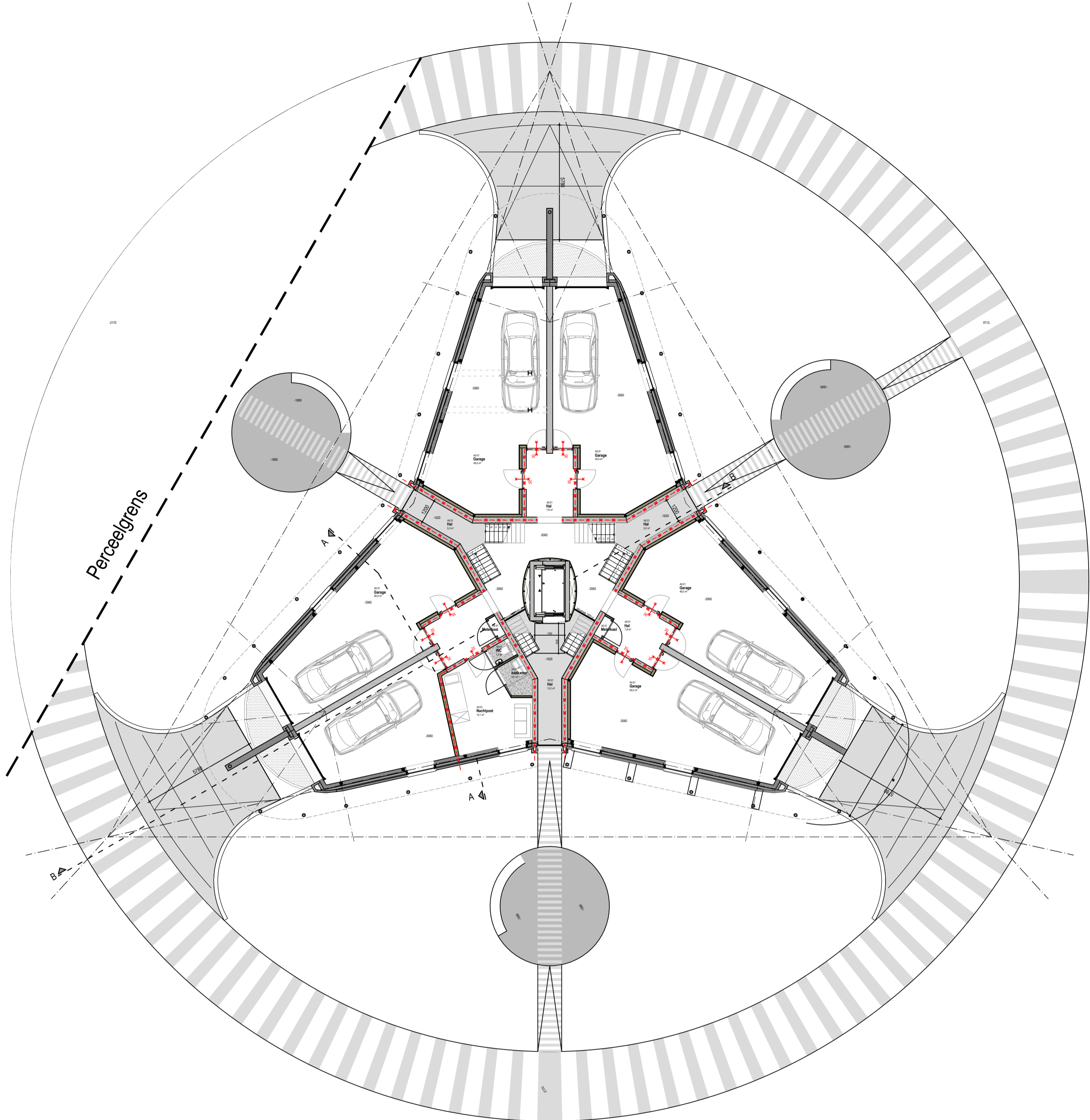
BEGANEGROND
