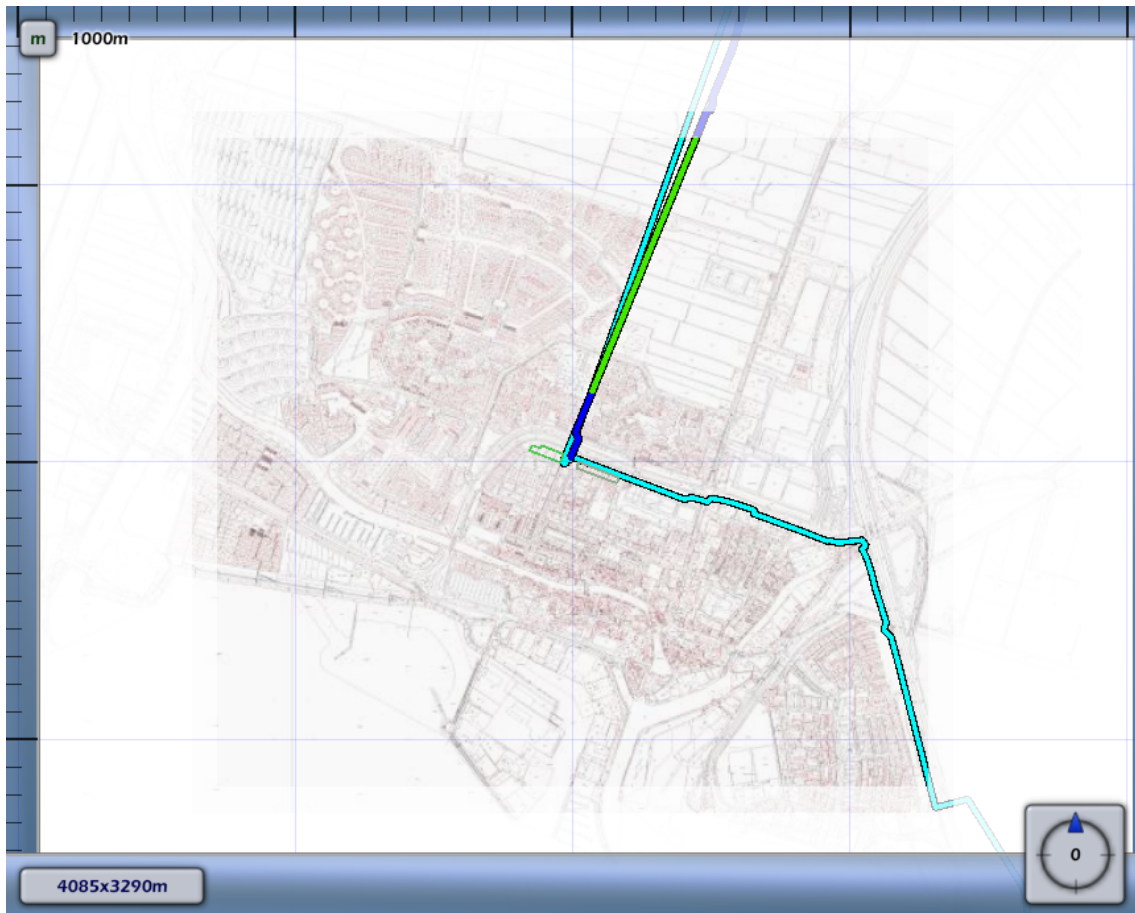
4.3 Figuur 4.3 Groepsrisico screening voor N-501-41 van N.V. Nederlandse Gasunie
