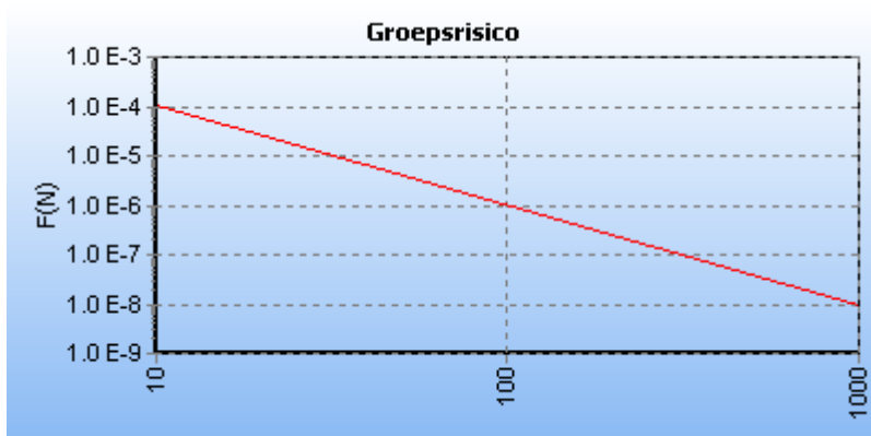
5.2 Figuur 5.2 FN curve voor N-501-26 van N.V. Nederlandse Gasunie voor de kilometer tussen stationing 12440.00 en stationing 13440.00
