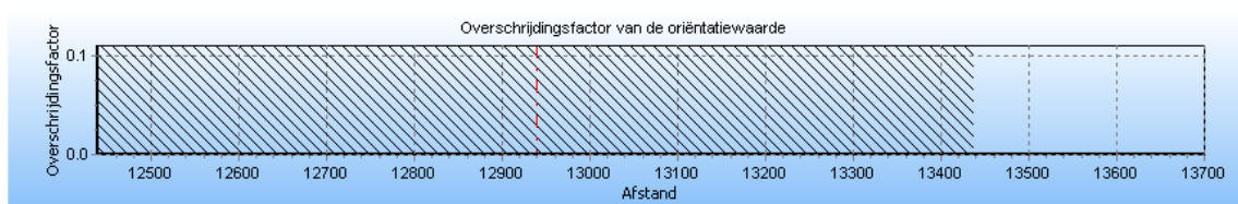
4.2 Figuur 4.2 Groepsrisico screening voor N-501-26 van N.V. Nederlandse Gasunie
