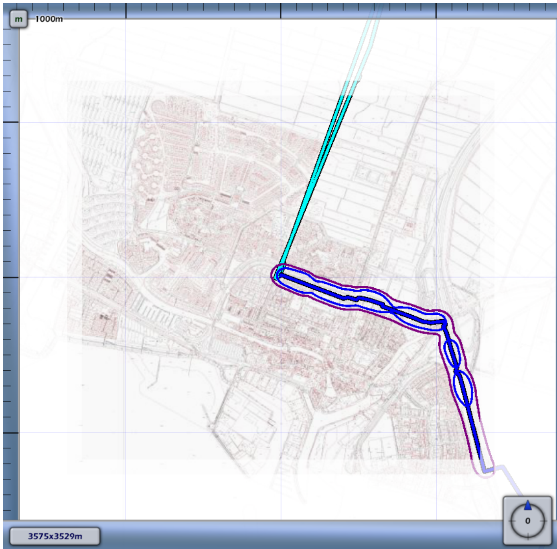
3.1 Figuur 3.1 Plaatsgebonden risico voor N-501-25 van N.V. Nederlandse Gasunie
