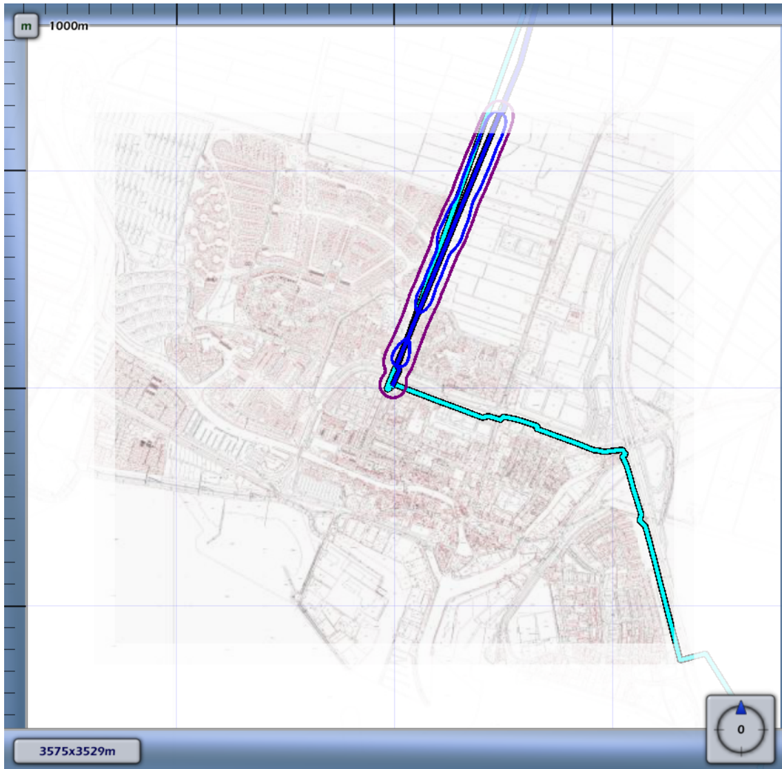
3.2 Figuur 3.2 Plaatsgebonden risico voor N-501-26 van N.V. Nederlandse Gasunie
