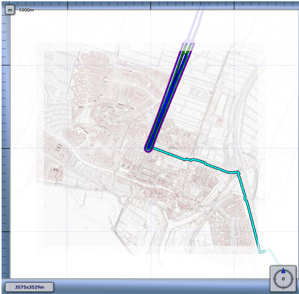
3.3 Figuur 3.3 Plaatsgebonden risico voor N-501-41 van N.V. Nederlandse Gasunie
