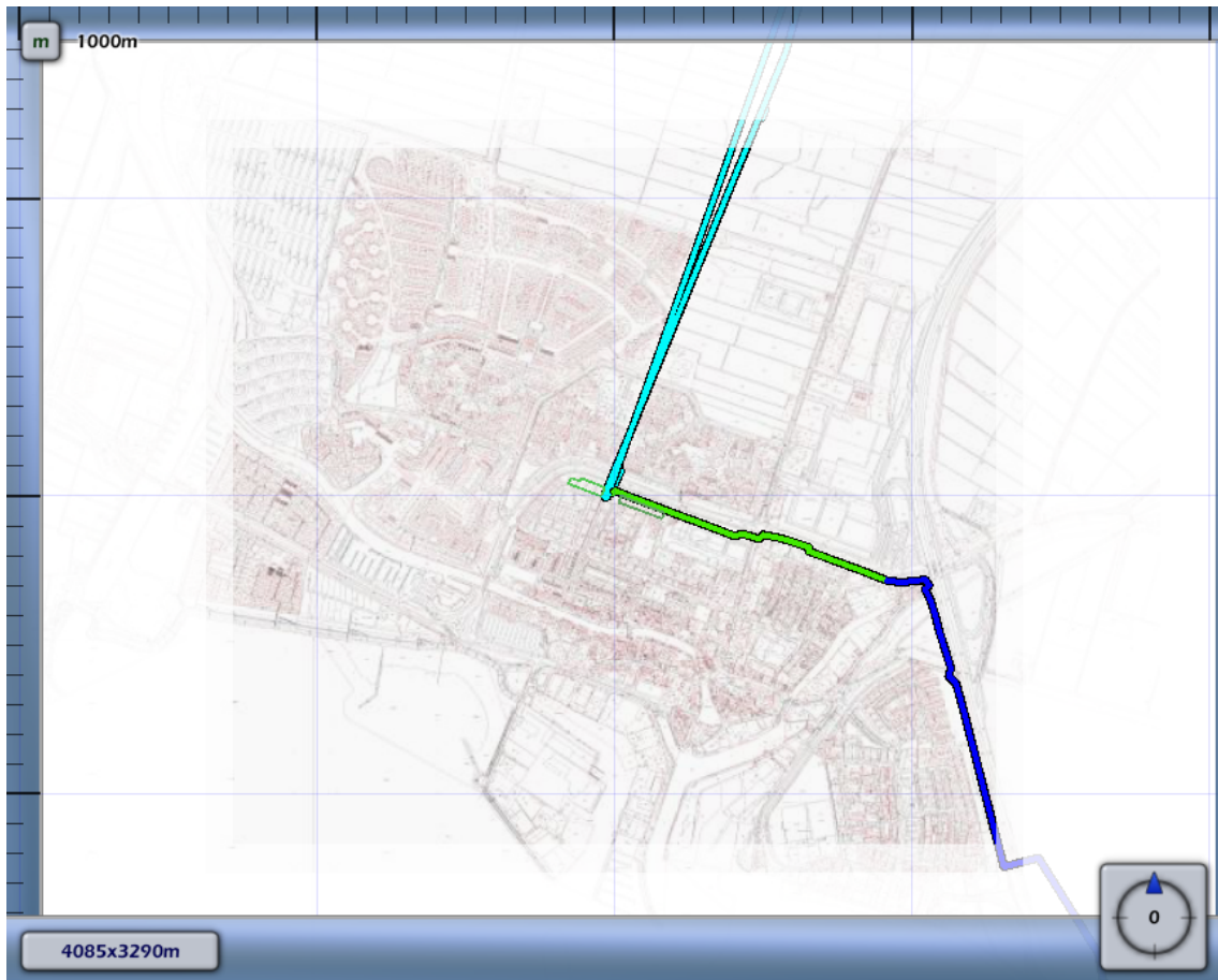
4.2 Figuur 4.2 Groepsrisico screening voor N-501-26 van N.V. Nederlandse Gasunie
