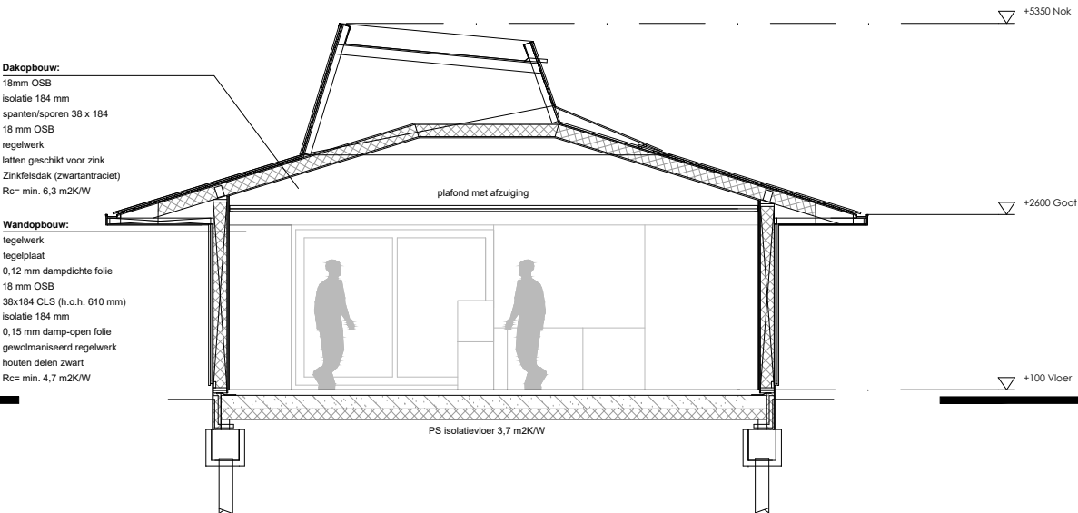
LANGSDOORSNEDE A - A
