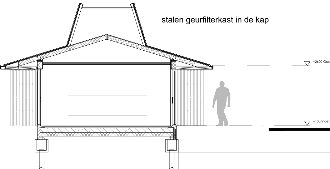
DWARSDOORSNEDE B - B
