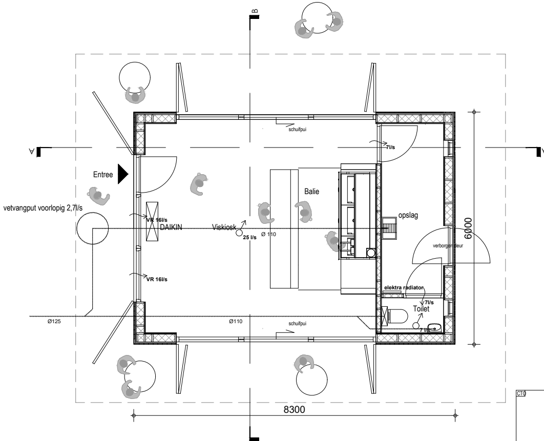
PLATTEGROND
