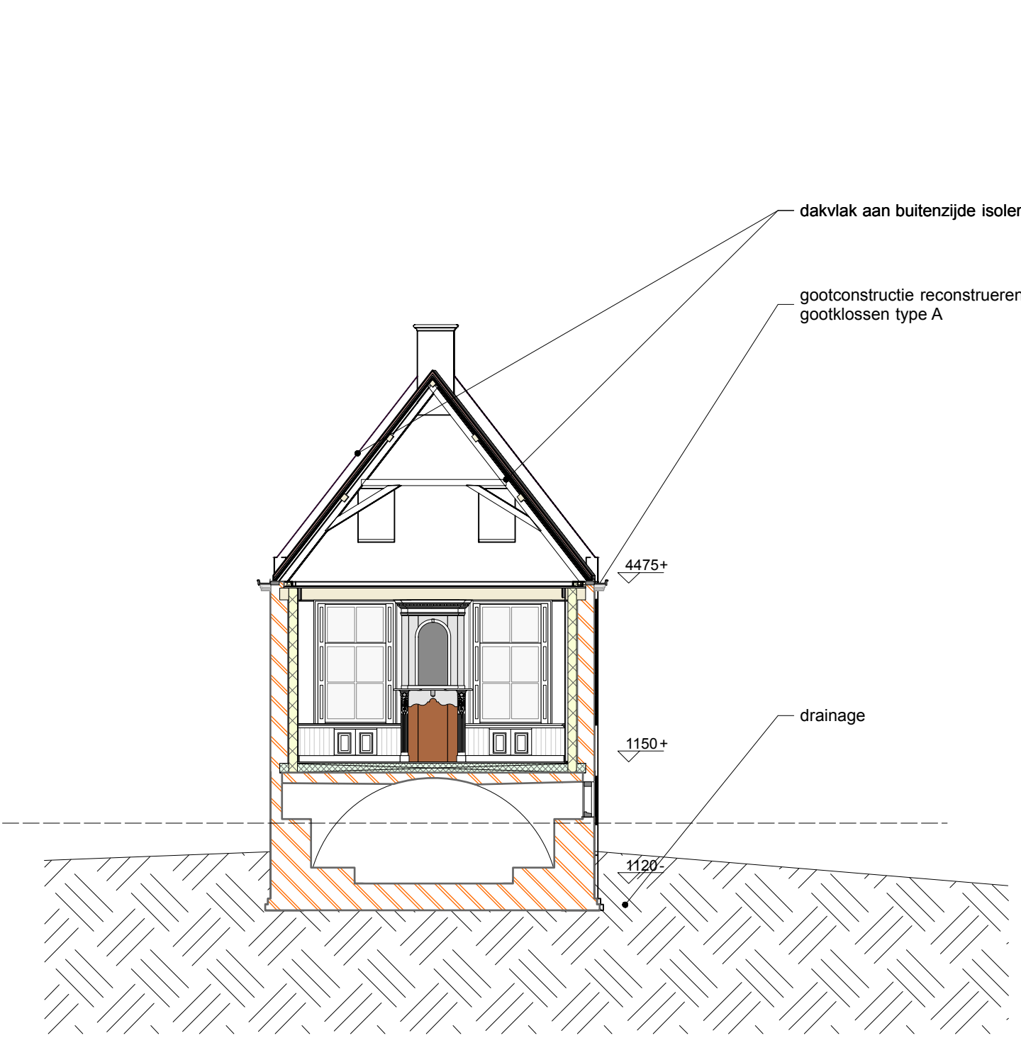
DOORSNEDE G-G
