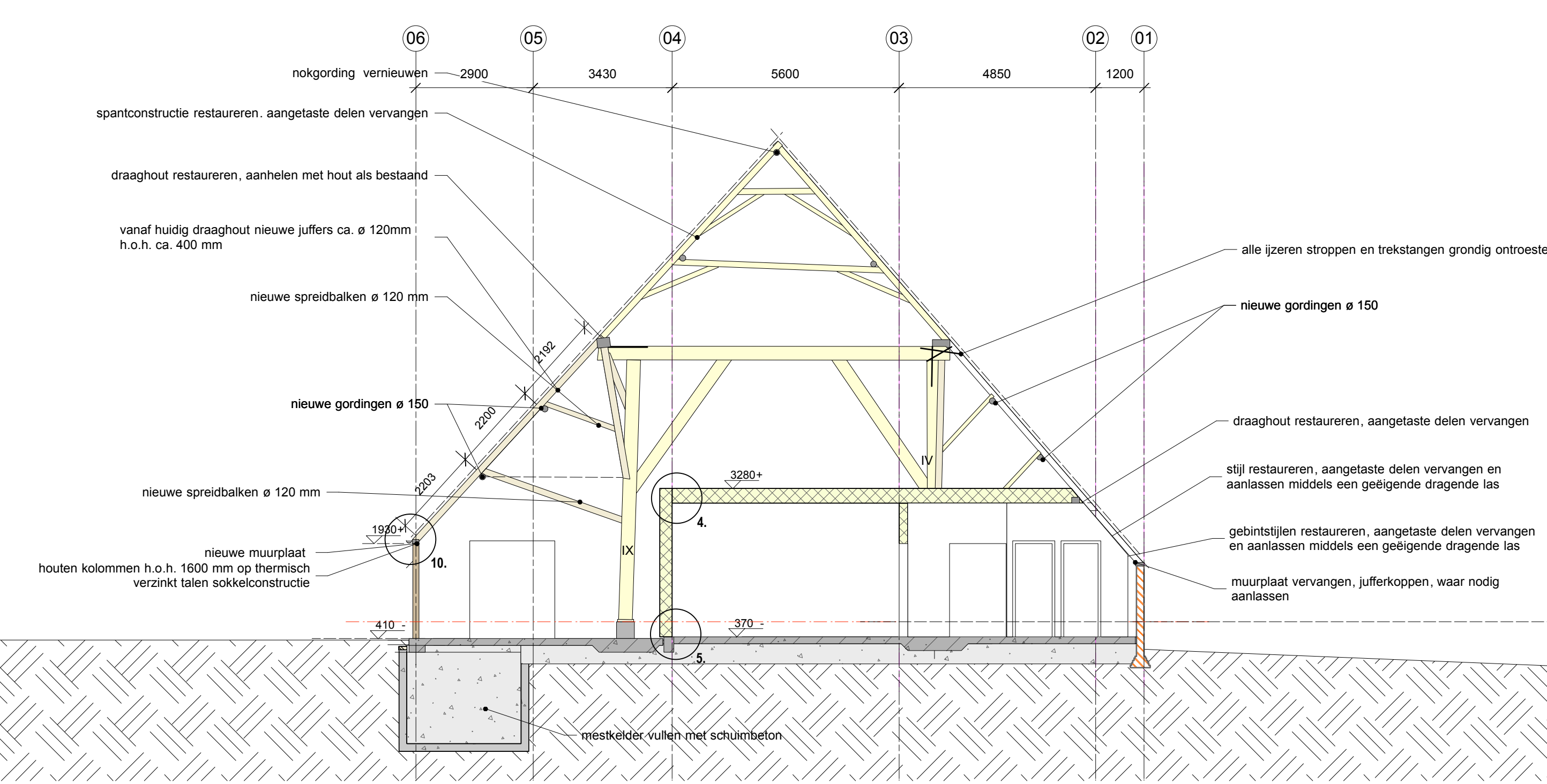
DOORSNEDE A-A
