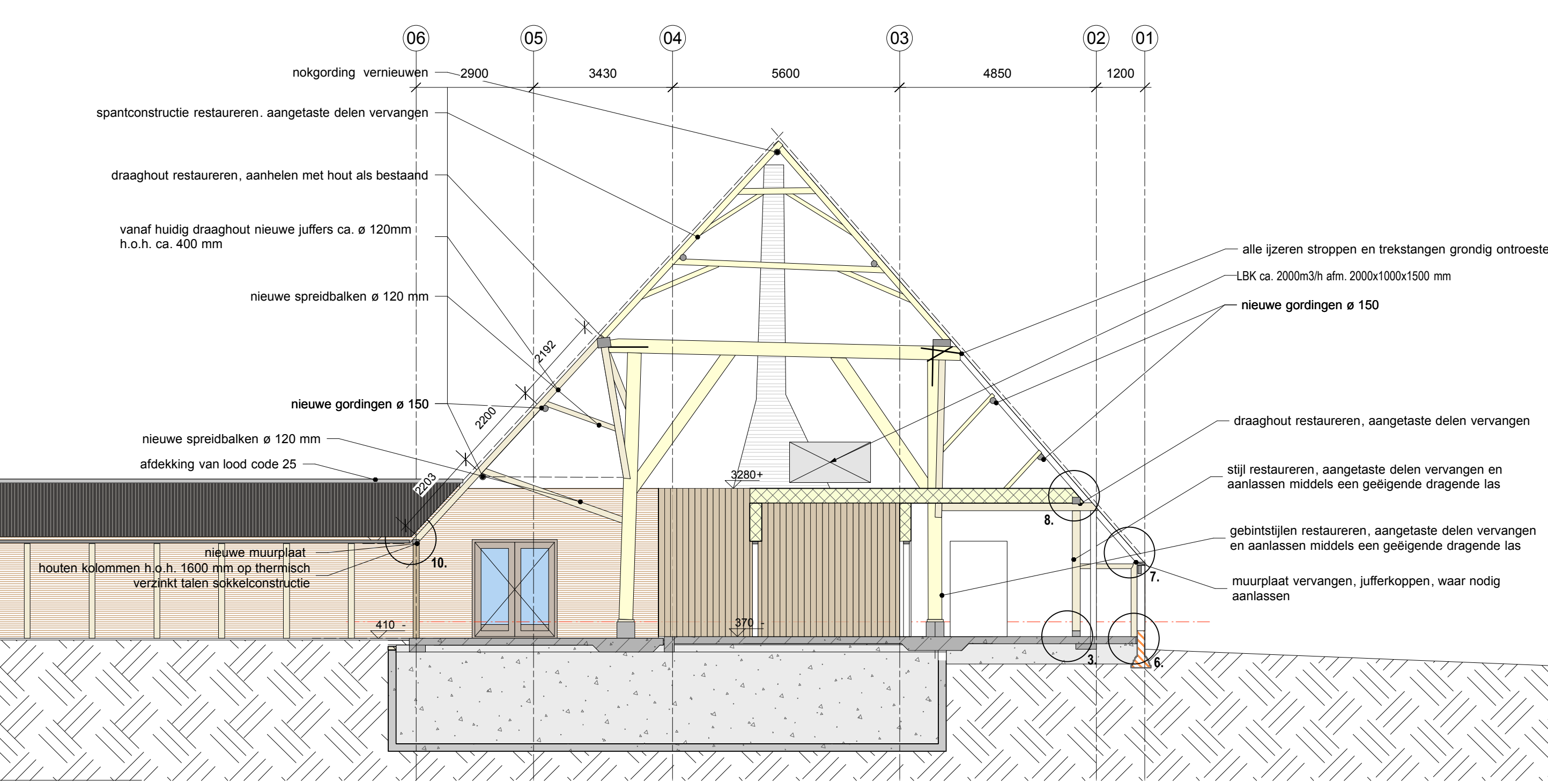
DOORSNEDE C-C
