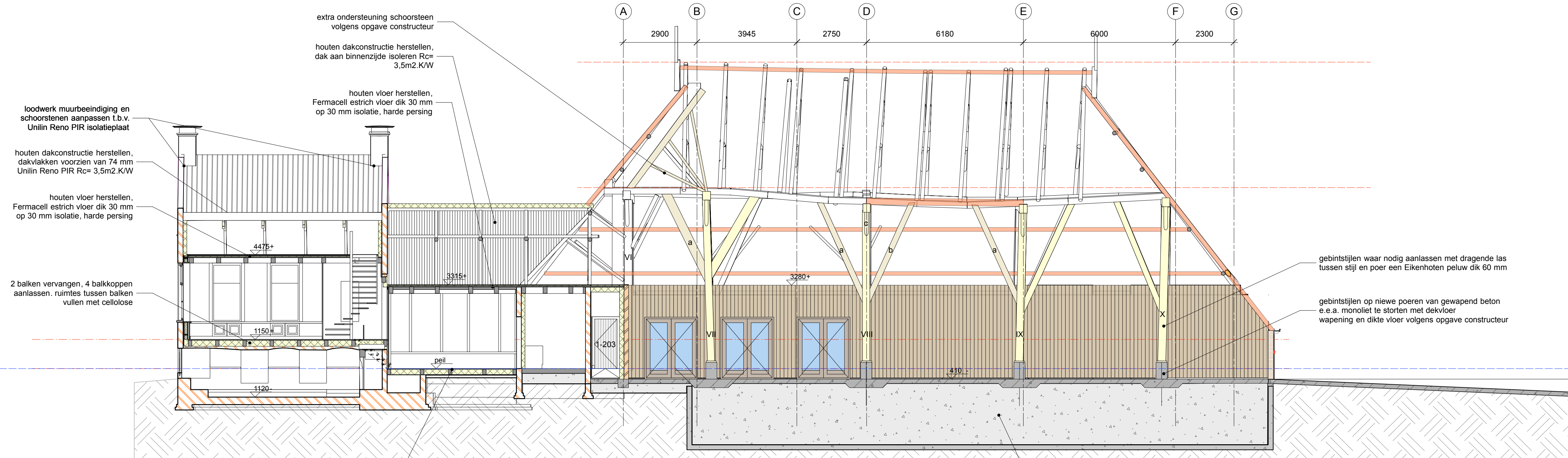
DOORSNEDE B-B
