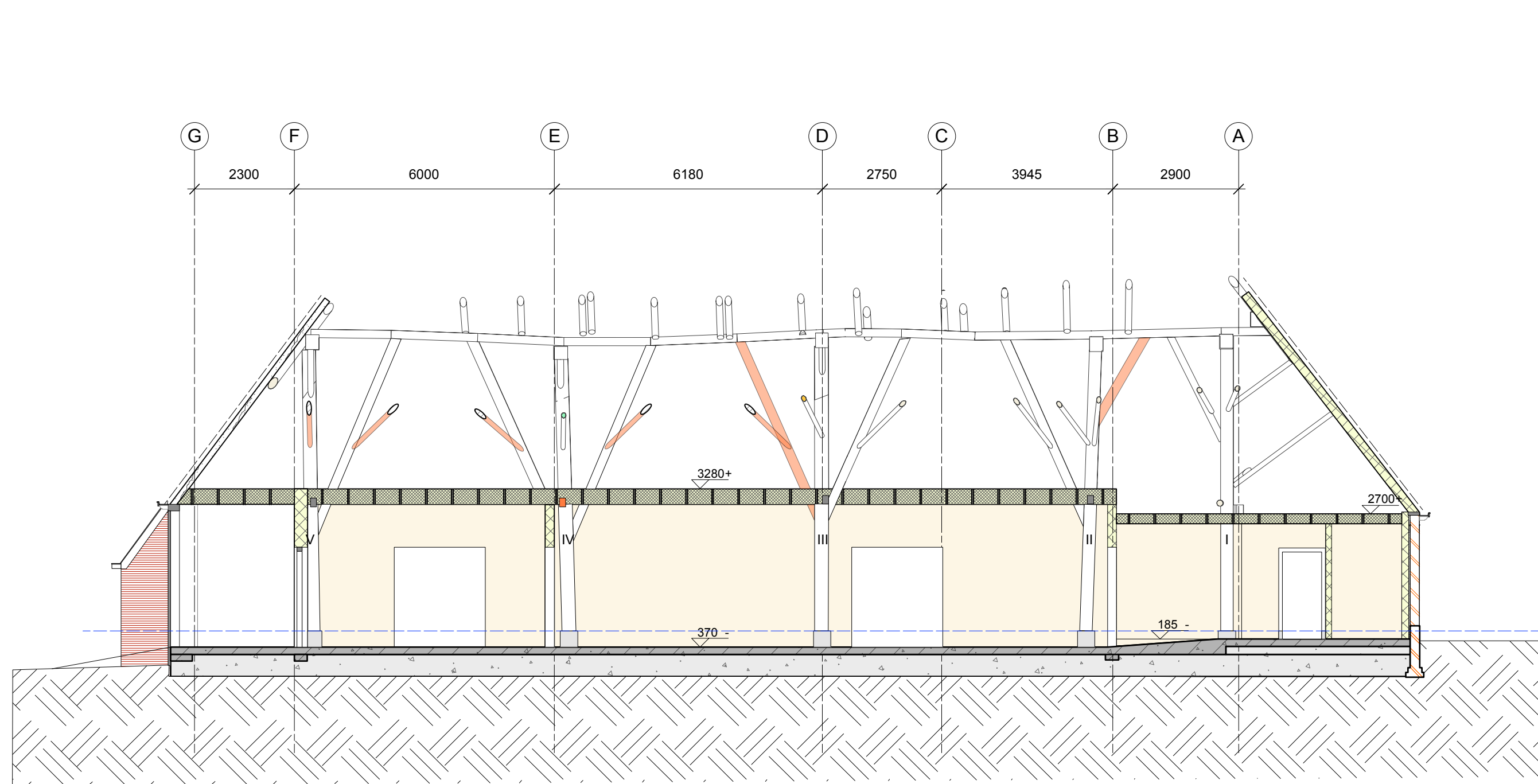
DOORSNEDE A-A
