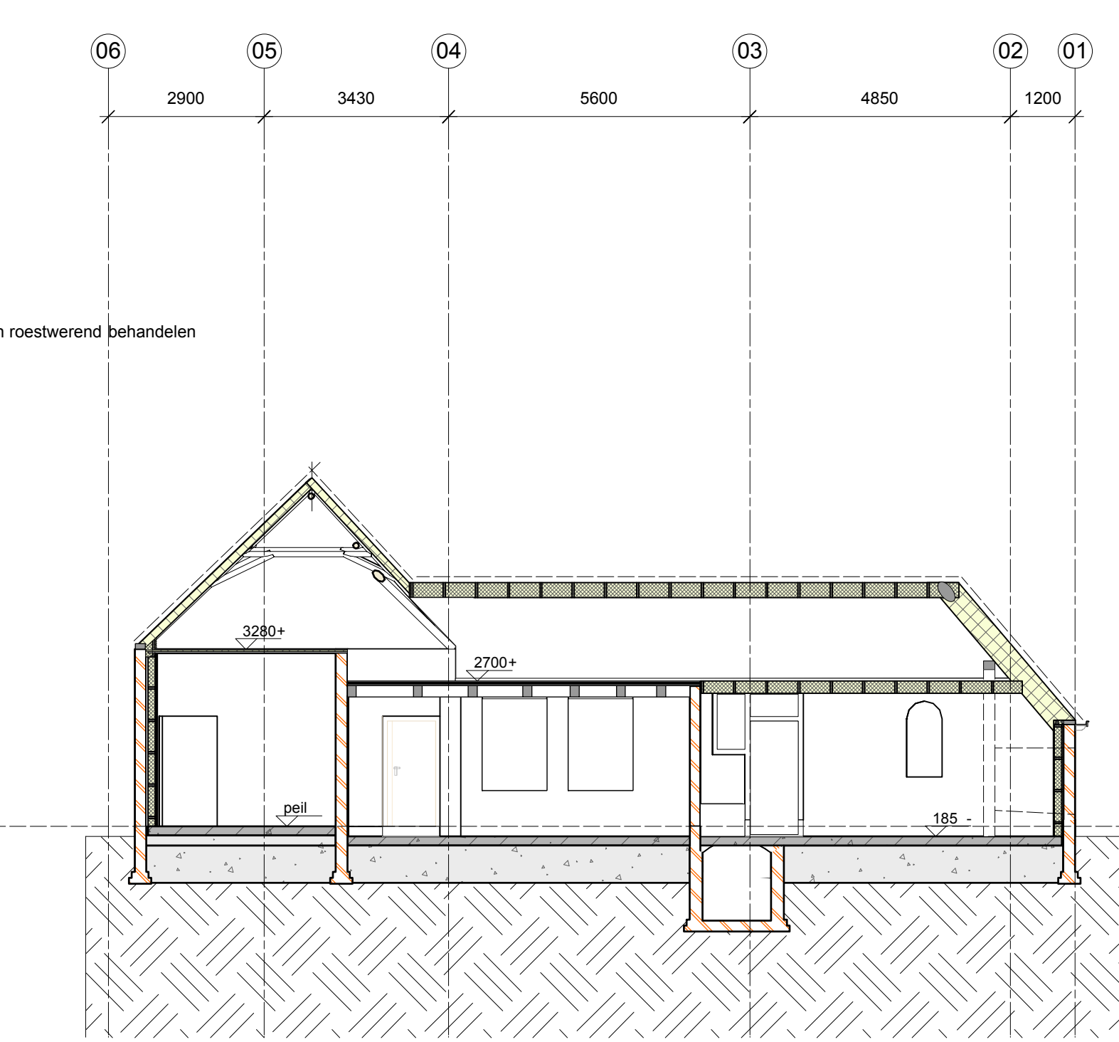
DOORSNEDE E-E
