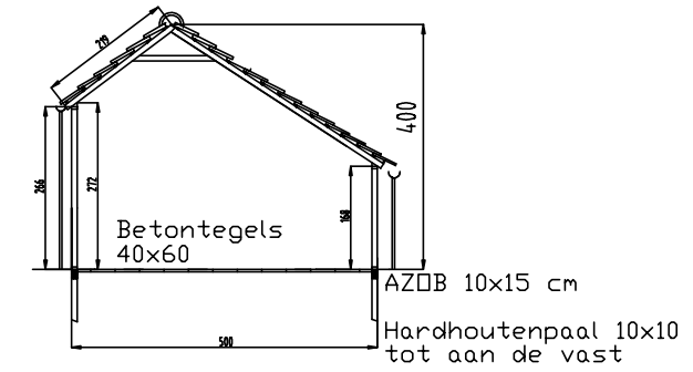
Doorsnede A - A
