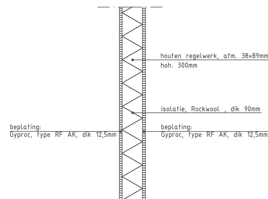
Detail A (schaal 1:10)
