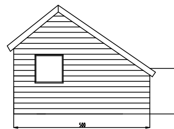
Linkerzijkant kapschuur
