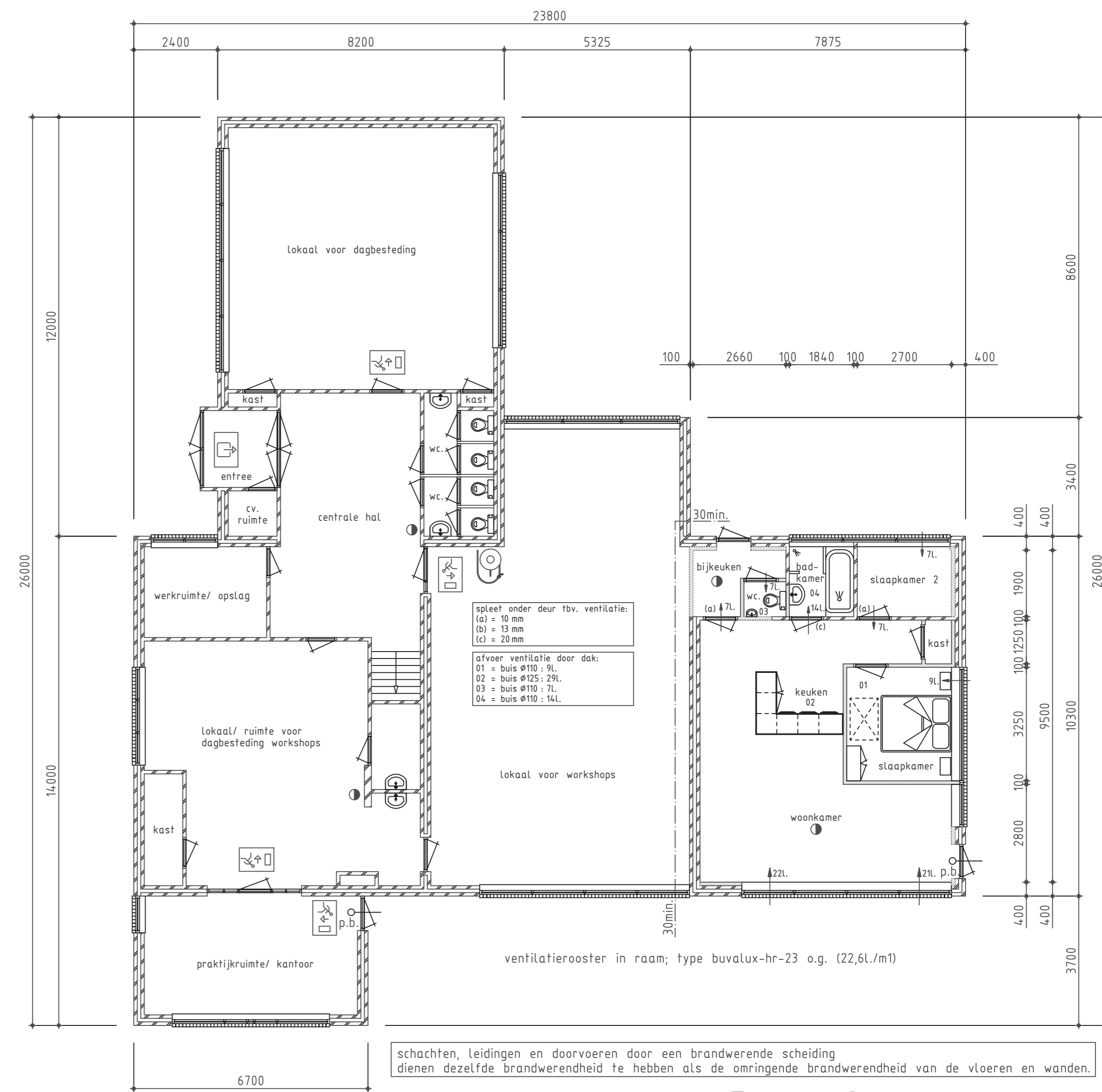
Beganeground Nieuw
