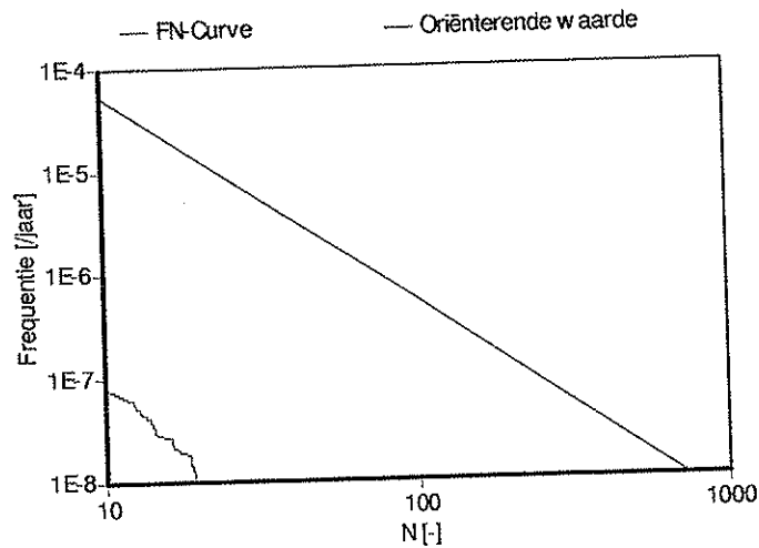
Figuur 2: FN-curve van leiding N-500-08-KR-001, de oriënterende waarde is anders dan gebruikelijk i.v.m. de lengte van de leiding, 550 meter.
