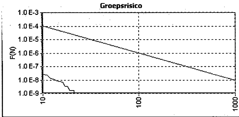
5.9 Figuur 5.9 FN curve voor N-579-01 van N.V. Nederlandse Gasunie voor de kilometer tussen stationing 3580.00 en stationing 4580.00
