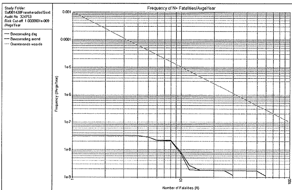
Figuur 5. Groepsrisico LPG-tankstation doorzet van 500 m 3 /jr tankauto voorzien van hittewerende coating
