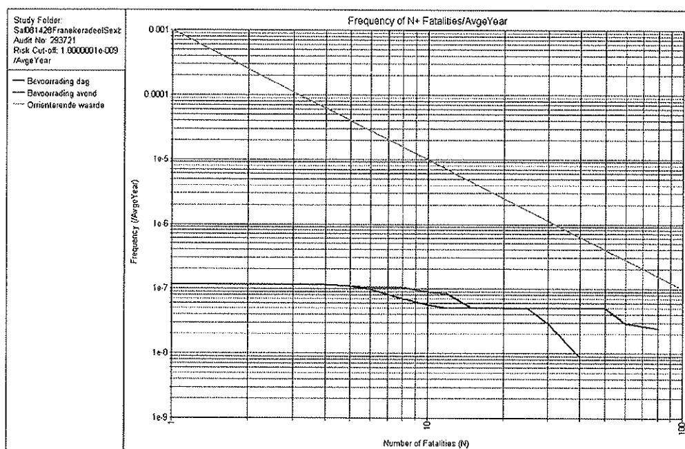
Figuur 2. Groepsrisico LPG-tankstation doorzet van 1000 m 3 /jr
