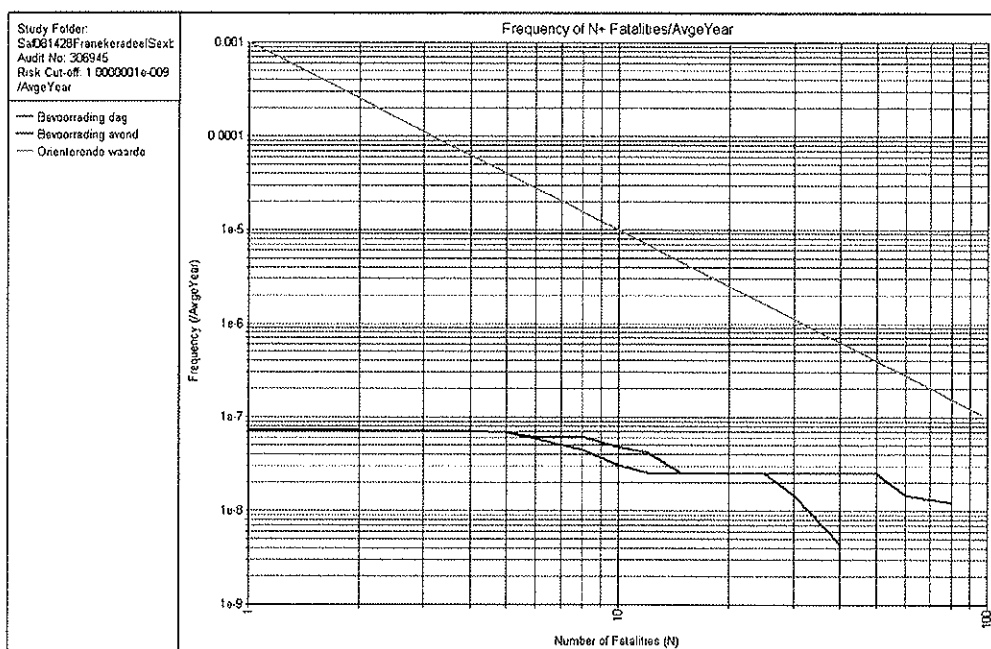
Figuur 4. Groepsrisico LPG-tankstation doorzet van 500 m 3 /jr
