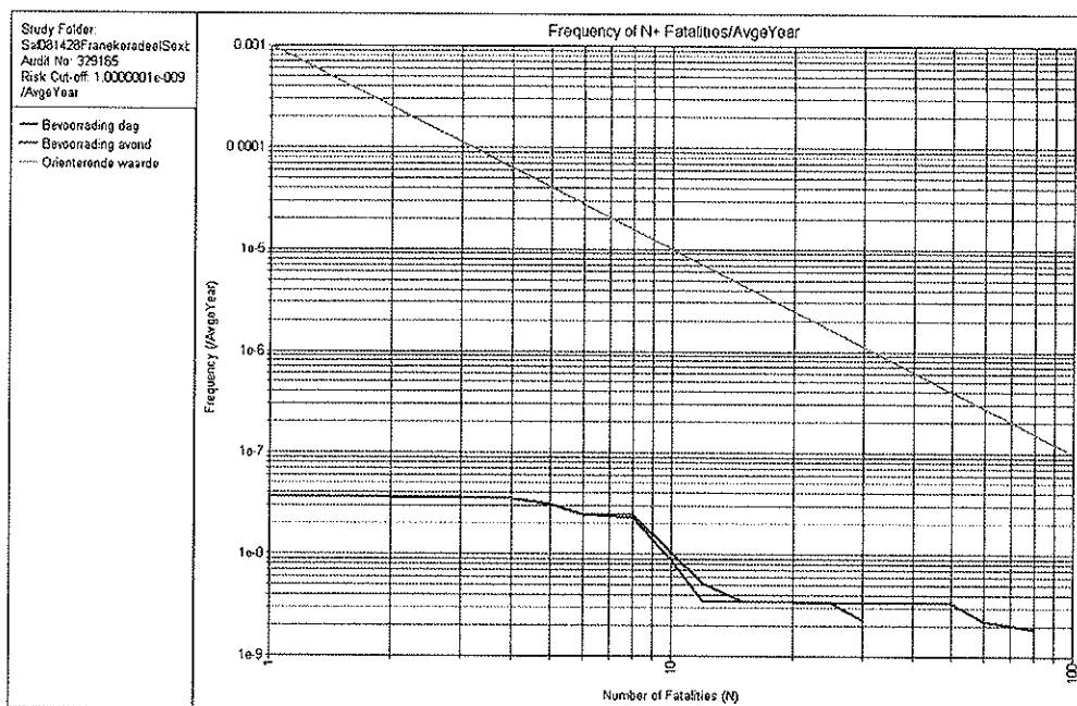
Figuur 3. Groepsrisico LPG-tankstation doorzet van 1000 m 3 /jr tankauto voorzien van hittewerende coating
