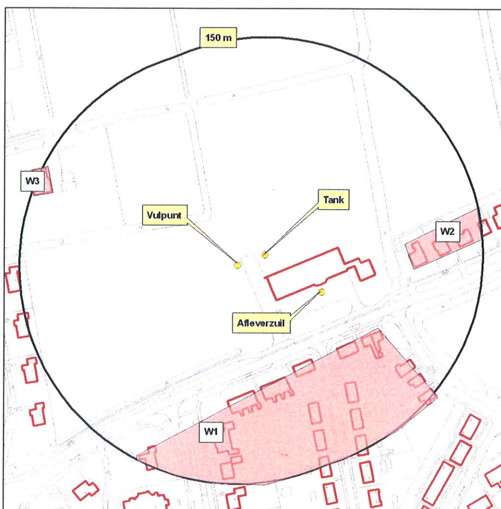
Figuur 1. Omgeving LPG-tankstation
