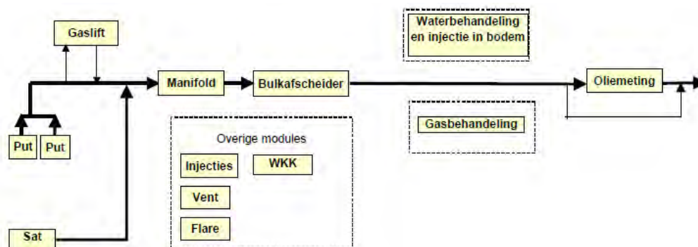
Figuur 3.2: Oliebehandelingsproces.
