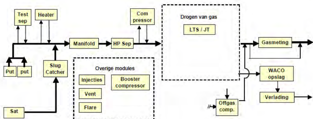
Figuur 3.1: Gasbehandelingsproces.
