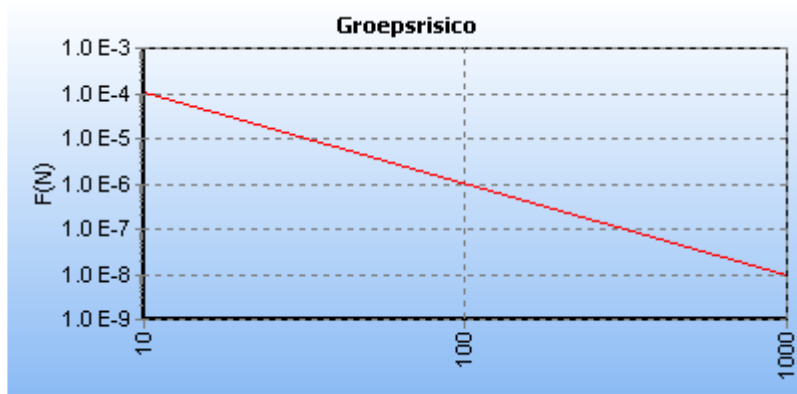
5.3 Figuur 5.3 FN curve voor N-505-07 van N.V. Nederlandse Gasunie voor de kilometer tussen stationing 0.00 en stationing 30.00
