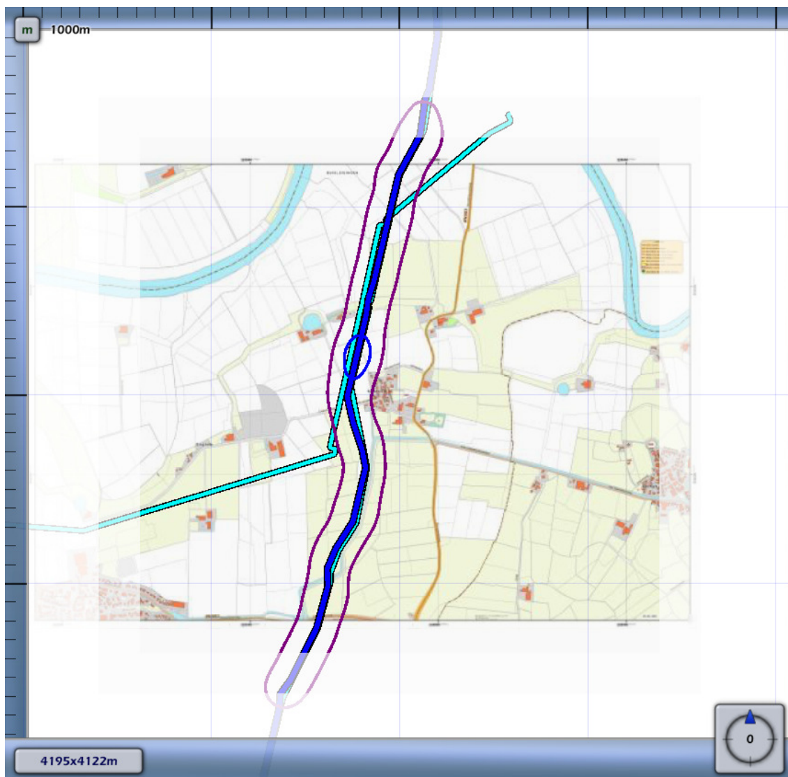
3.2 Figuur 3.2 Plaatsgebonden risico voor A-606 van N.V. Nederlandse Gasunie
