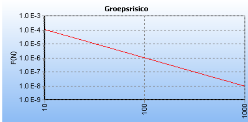
5.4 Figuur 5.4 FN curve voor {5CD41B32-CB71-49BC-9F40-D5BF8E7EBE5D}_000141 van Nederlandse Aardolie Maatschappij BV voor de kilometer tussen stationing 8560.00 en stationing 9560.00
