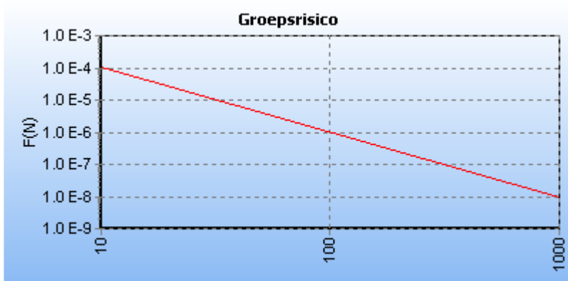
5.2 Figuur 5.2 FN curve voor A-606 van N.V. Nederlandse Gasunie voor de kilometer tussen stationing 13860.00 en stationing 14860.00
