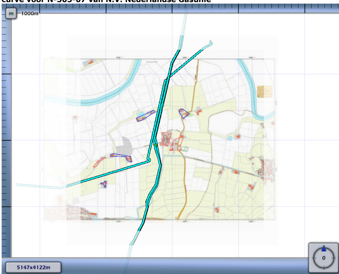
Figuur 4.3 Kilometer leiding behorende bij de maximale overschrijding van de FN-curve voor N-505-07 van N.V. Nederlandse Gasunie
