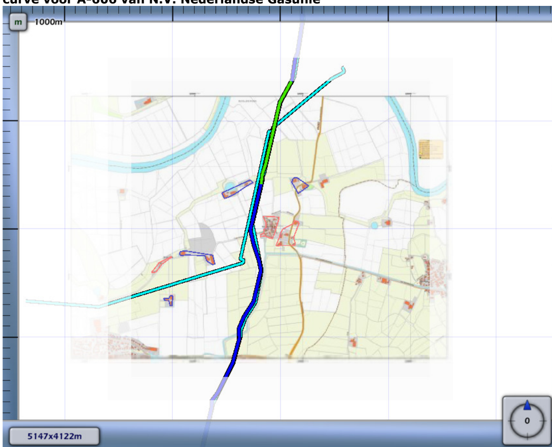
Figuur 4.2 Kilometer leiding behorende bij de maximale overschrijding van de FN-curve voor A-606 van N.V. Nederlandse Gasunie
