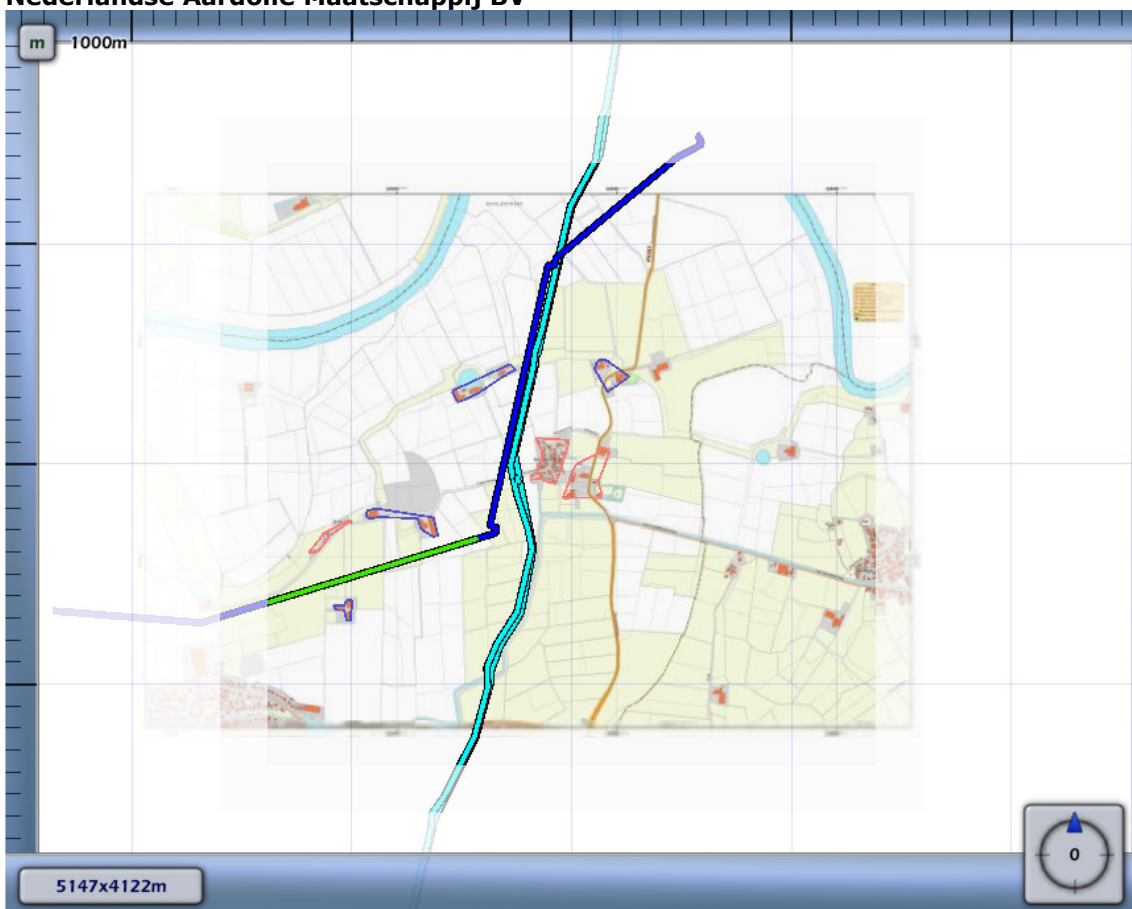
Figuur 4.4 Kilometer leiding behorende bij de maximale overschrijding van de FN-curve voor {5CD41B32-CB71-49BC-9F40-D5BF8E7EBE5D}_000141 van Nederlandse Aardolie Maatschappij BV
