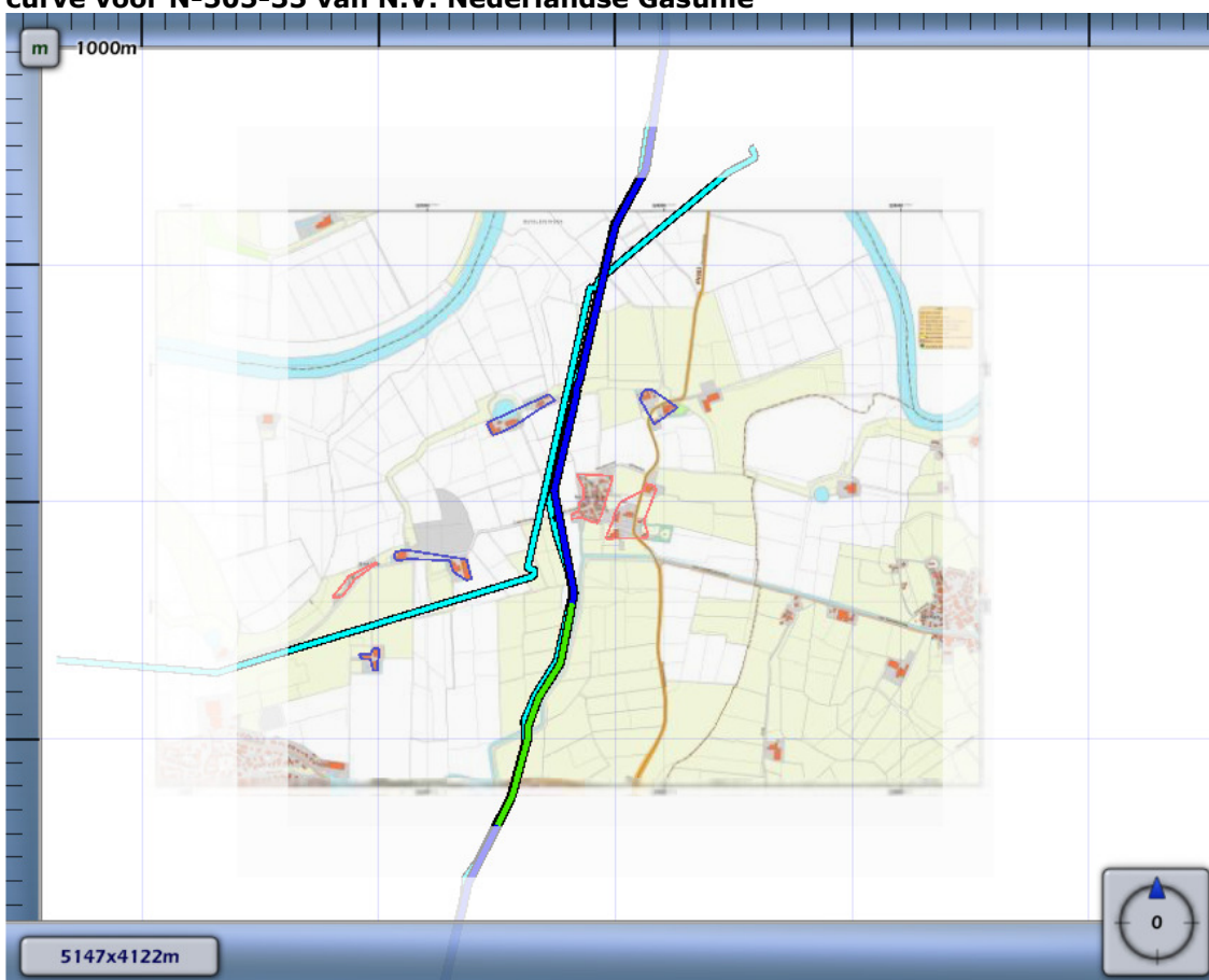
Figuur 4.1 Kilometer leiding behorende bij de maximale overschrijding van de FN-curve voor N-505-35 van N.V. Nederlandse Gasunie
