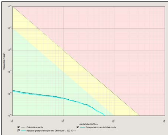
fN-curve toekomstige situatie (dd. 7-12-2012)
